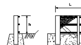
落石防護工
