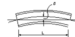
桁製作工(主桁、主構のそり)
