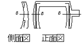
鋼製橋脚製作工(仮組立時)(おのりキャバー及び柱の曲がり)
