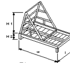
図d 鋼製スリットダム 鋼製堰堤本体工(透過型)(図d)
