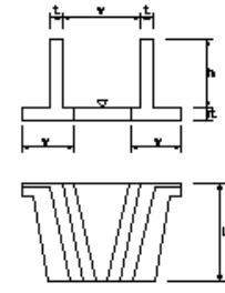
水叩工
