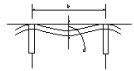
桁製作工(仮組立による検査を省略する場合)(板の平面度)
