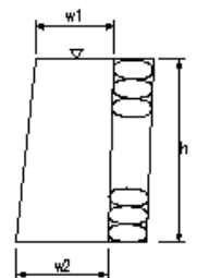
取付擁壁工(3)
