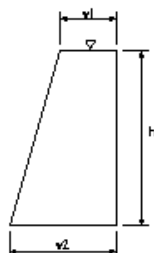
小型擁壁工
