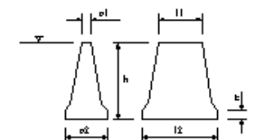
RC躯体工(重力式)(半重力式)
