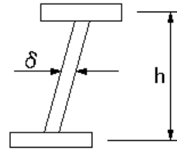
桁製作工(主げた、主構の鉛直度)
