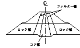
コアの盛立
