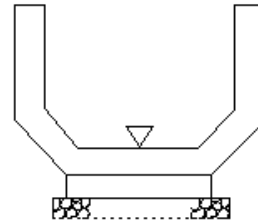
側溝工(グレキャストU型側溝工)
