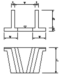
翼壁工
