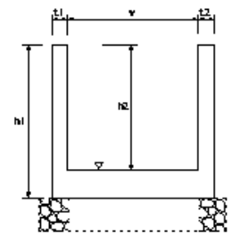
堤脚水路工
