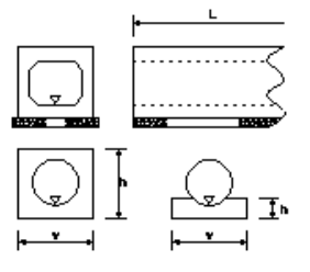
樋門接続暗渠工
