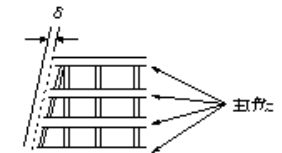
横断歩道橋製作工(主けた、主構の橋端における出入差)
