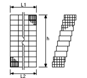
ふとんかご、かご枠
