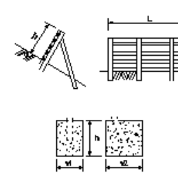
雪崩予防柵工
