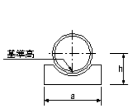
管渠工(開削工法)
