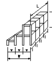
図a 格子形鋼製砂防ダム
