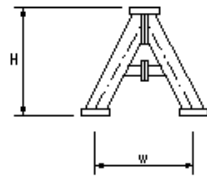
図b 鋼製スリットダムA型 鋼製堰堤製作工(仮組立時)(図b)
