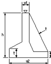
取付擁壁工(5)
