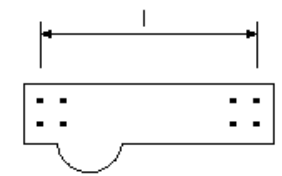
桁製作工(部材長)(鋼けた)
