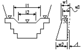
鋼製堰堤本体工(不透過型)
