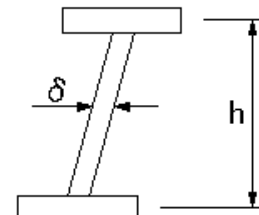
桁製作工(主げた、主構の鉛直度)
