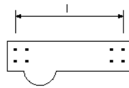
桁製作工(部材長)(鋼けた)
