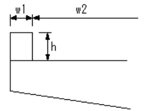
地覆工
