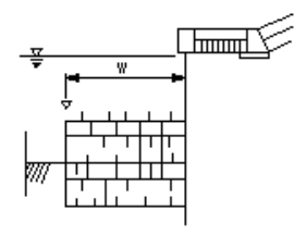
沈床工
