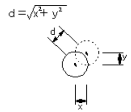
既製杭工
