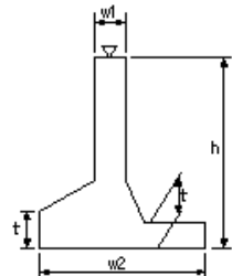
取付擁壁工(4)
