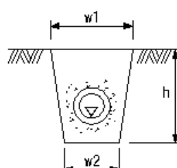
暗渠工
