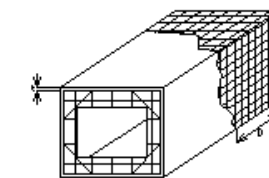
鉄筋の組立て
