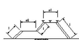
路体盛土工・路床盛土工・軽量盛土工
