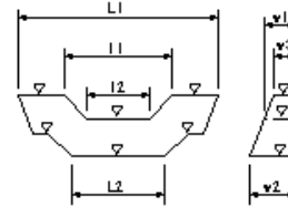
コンクリート堰堤本体工 コンクリート副堰堤工
