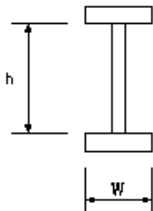
I型プレートガーター
