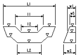
床固め本体工
