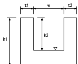
山腹集水路・排水路工
