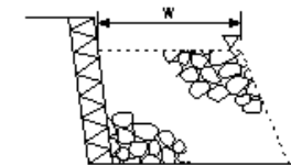
捨石工
