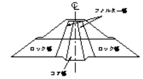
フィルターの盛立
