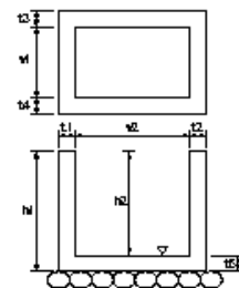
排水構造物修繕工(集水構工)
