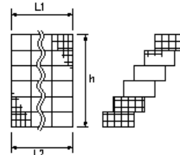
かご工(ふとんかご工)
