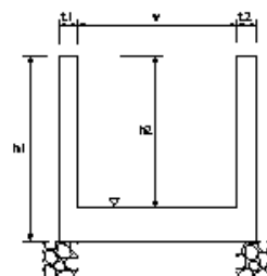
場所打水路工
