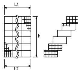
かご工(ふとんかご)
