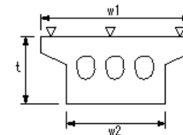
PCホロースラブ製作工
