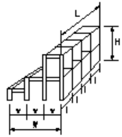
図a 格子形鋼製砂防ダム 鋼製堰堤製作工(仮組立時)(図a)
