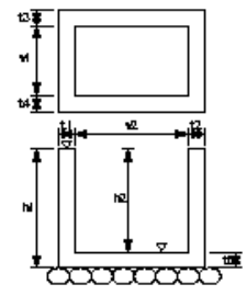
ハンドホール工
