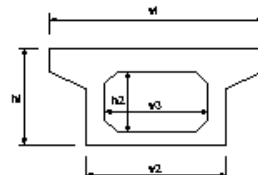
PC箱桁製作工
