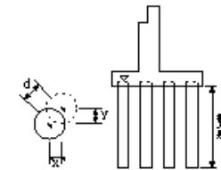
場所打杭工
