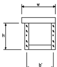
トラス弦材桁製作工(トラス・アーチ等)
