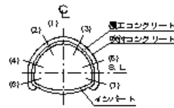
吹付工
