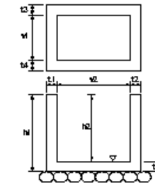
ケーブル配管工(ハンドホール)
