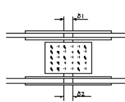
桁製作工(現場継手部のすき間)
