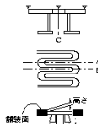
橋梁付属物工(鋼製フィンガージョイント)
