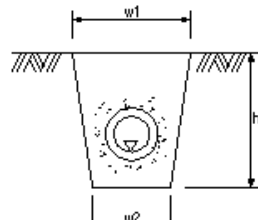
山腹暗渠工
