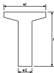
ポステンションT(①)桁製作工
