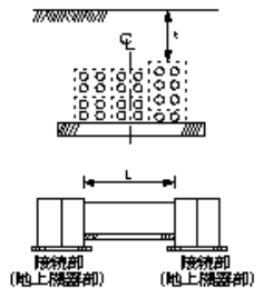
管路工
