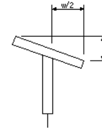
プレーム用桁製作工(フランジの直角度)
