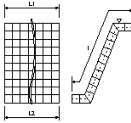
コンクリートブロック工(連節ブロック張り)*1
