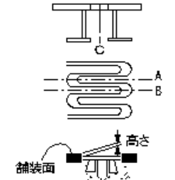
伸縮装置工(鋼製フィンガージョイント)
