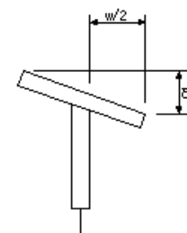
桁製作工(フランジの直角度)
