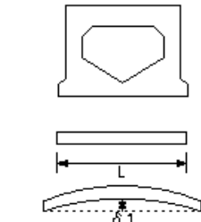
プレテンション桁製作工(購入工)スラブ桁
