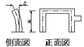
鋼製橋脚製作工(仮組立時)(柱の鉛直度)
