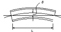
横断歩道橋製作工(主けた、主構のそり)
