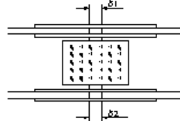
桁製作工(現場継手部のすき間)
