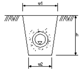
暗渠工
