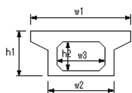
PC押し出し箱桁製作工
