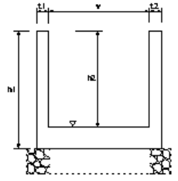
側溝工
