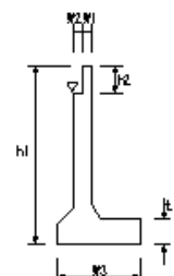
管理橋橋台工(4)
