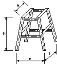
図c 鋼製スリットダムB型 鋼製堰堤製作工(仮組立時)(図c)
