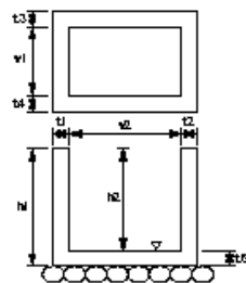
集水樹工
