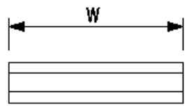
鋼製伸縮継手製作工(部材)
