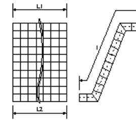
連節ブロック張り工
