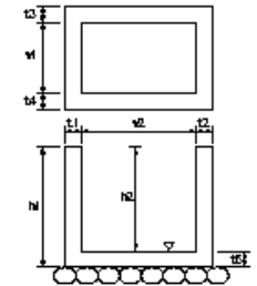
街渠樹・マンホール工(街渠樹工)(マンホール工)
