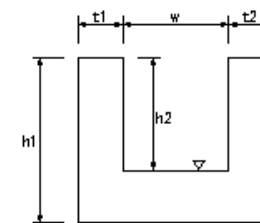
側溝工
