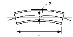
桁製作工(主げた、主構のそり)
