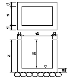
集水樹工
