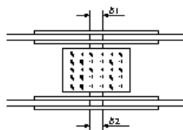
横断歩道橋製作工(現場継手部のすき間)
