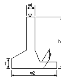
場所打擁壁工(4)
