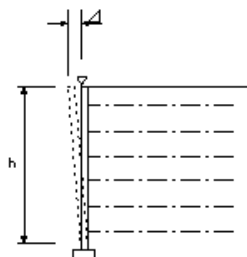
補強土壁工(補強土(テールアルメ)壁工法)(多数アンカー式補強土工法)
