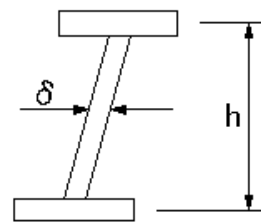
桁製作工(主げた、主構の鉛直度)
