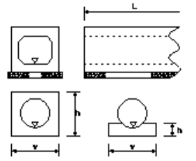
函渠工(PC函渠)
