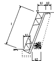
石積(長)工
