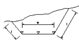
掘削工(切土工)
