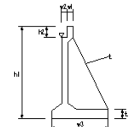
管理橋橋台工(2)
