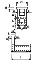
函渠工(本体工)
