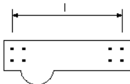
桁製作工(部材長)(鋼(げた))
