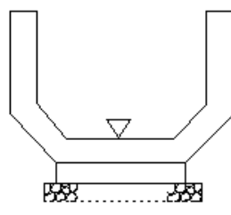
側溝工(プレキャストU型側溝)
