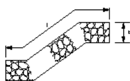
かご工(じゃかご)
