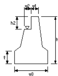
管理橋橋台工(1)
