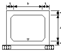
現場打水路
