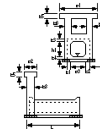
函渠工(本体工)
