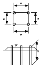
パチカルドレーン工(サンドドレーン工) (ベ ーパドレーン工)(袋詰式サンドドレーン工)
