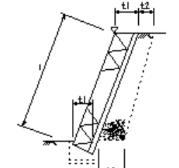
石積(石)工
