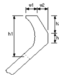
波返工
