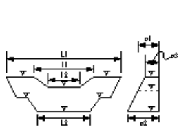
本体工(床固め本体工)
