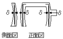
鋼製橋脚製作工(仮組立時)(はりのキャッチャー及び柱の曲がり)
