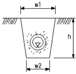
暗渠工
