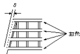
横断歩道橋製作工(仮組立による検査を省略する場合)(主桁、主構の橋端における出入差)
