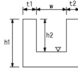
魚道工*1
