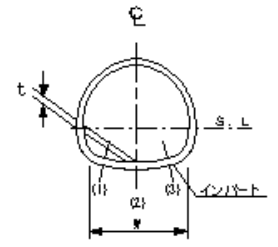
インパート本体内工
