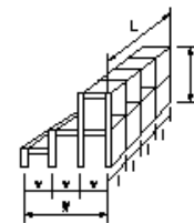
図a 格子形鋼製砂防ダム 鋼製堰堤本体内工(透過型)(図a)
