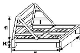
図d 鋼製L型 スリットダム 鋼製堰堤本体内工(透過型)(図d)
