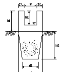
山腹明暗渠工
