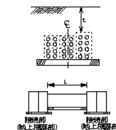
管路工
