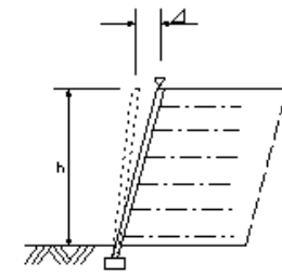
補強土壁工(ワイヤーウォール工法)
