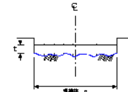
切削オーバーレイ工
