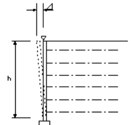
補強土壁工・ジオブロック工法
