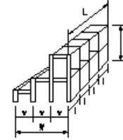
図a 格子形鋼製砂防ダム 鋼製ダム本体内工(透過型)(図a)
