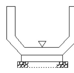
プレキャストカルバート工(プレキャストブロック工) プレキャストカルバート工(プレキャストパイプ工) 側溝工(プレキャストU型側溝) (コルゲートフルーム) (自由勾配側溝)
