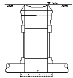
小型マンホール工
