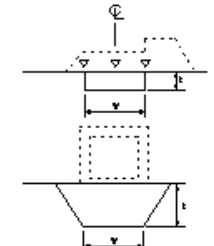
置換工
