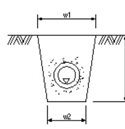
暗渠工
