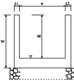
側溝工
