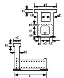
函渠工(本体工)*1
