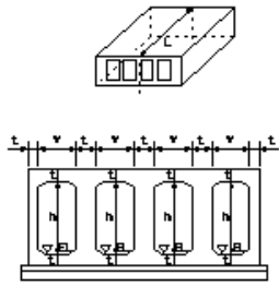
現場打ちボックス工
