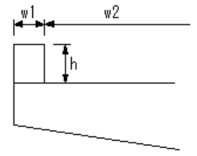
地覆工
