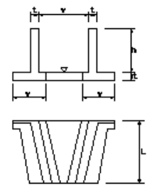
翼壁工
