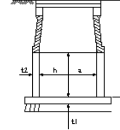
標準人孔築造工
