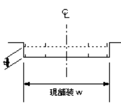
路面切削工
