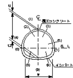
インパート本体内工
