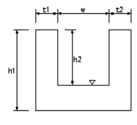
魚道本体工
