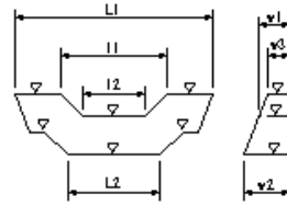
床固め本體工
