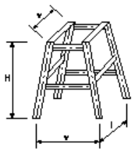
図c 鋼製スリットダムB型 鋼製堰堤本体内工(透過型)(図c)
