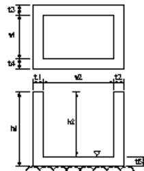
集水樹工
