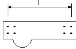
桁製作工(部材長)(プレートガーター)
