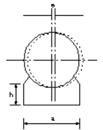
開削管渠工
