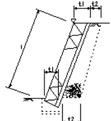
石積(張)工
