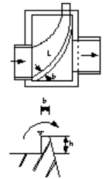
越流堰(雨水吐室)
