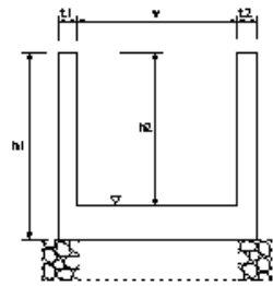
堤脚水路工
