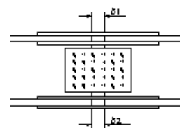
桁製作工(仮組立による検査を省略する場合)(現場継手部のすき間)
