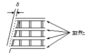
桁製作工(仮組立による検査を省略する場合)(主桁、主構の橋端における出入り差)
