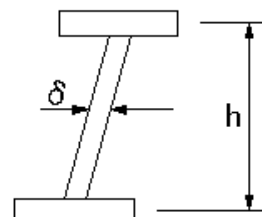
桁製作工(仮組立による検査を省略する場合)(主桁、主構の鉛直度)
