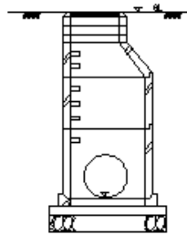
組立マンホール工
