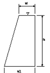
コンクリート擁壁工(1)
