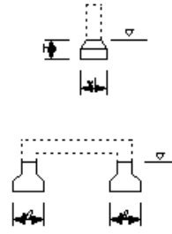
橋脚フーチング工(門型)
