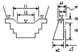
鋼製ダム本体内工(不透過型)8/1/7/5/1
