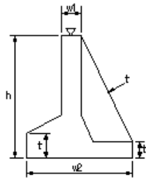
取付擁壁工(5)
