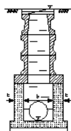
標準マンホール工
