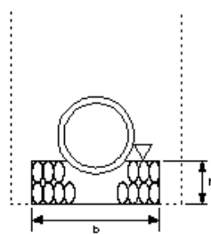
碎石基礎
