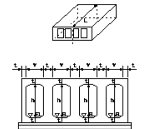
現場打ちボックス工
