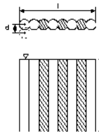
地中連続壁工(柱列式)1
