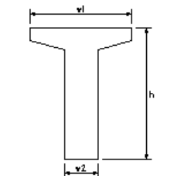
ポストテンションT(D)桁製作工
