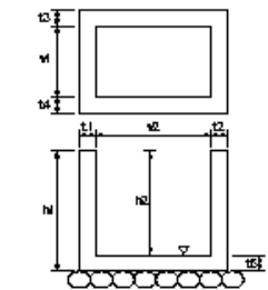
集水樹工
