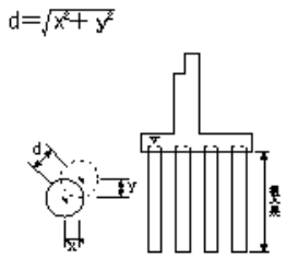
既製杭工
