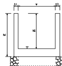
堤脚水路工
