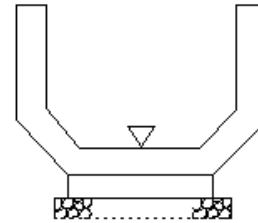
側溝工(プレキャストU型側溝工)
