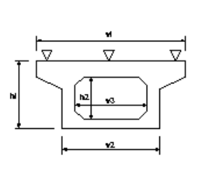
PC箱桁製作工・PC片持箱桁製作工
