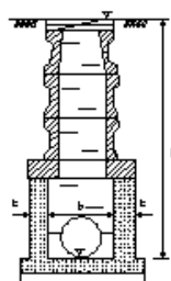
12/1/7標準マンホール工
