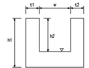
山腹集水路・排水路工
