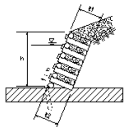
木製護岸工
