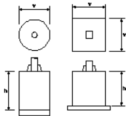
照明工(照明柱基礎工)
