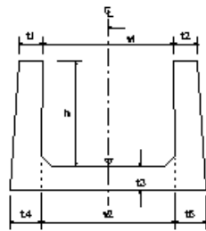
本体工(余水吐工)
