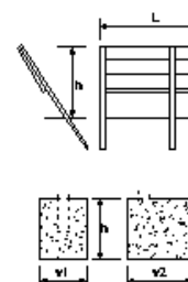
防雪柵工
