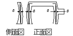
鋼製橋脚製作工(仮組立時)(仮りのキャンバー及び柱の曲がり)
