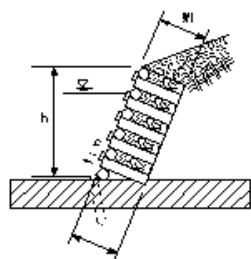
木製護岸工27/2/3/6
