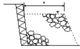
捨石工
