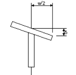
桁製作工(フランジの直角度)
