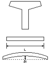
プレテンション筋購入工(けた橋)
