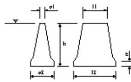
RC躯体工(重力式)(半重力式)
