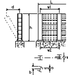
遮音壁本体工(1)
