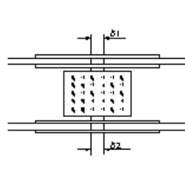
桁製作工(現場継手部のすき間)
