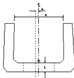
二次製品水路工(L型、大型水路)
