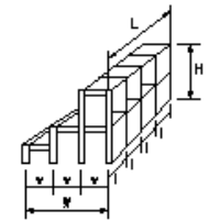
図a 格子形鋼製砂防ダム
