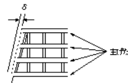
桁製作工(仮組立による検査を省略する 場合)(主桁、主構の橋端における出入り)
