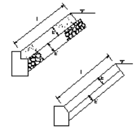
護岸工_コンクリート被覆工
