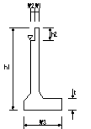
管理橋橋台工(4)
