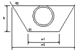
砂基礎工
