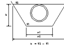
21/1/4/2砂基礎工
