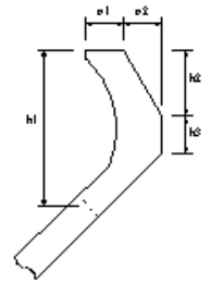
波返工
