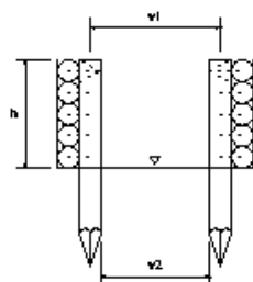
木製流路工
