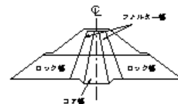
フィルターの盛立
