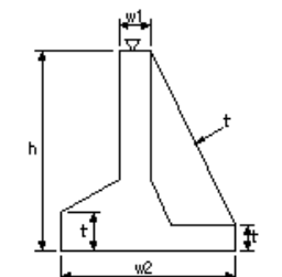
コンクリート擁壁工(5)
