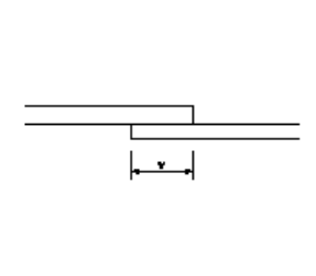
防水工(防水)
