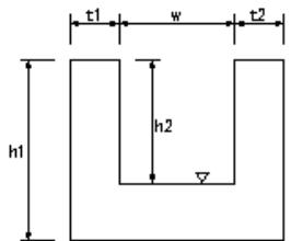
側溝工
