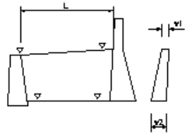
側壁工
