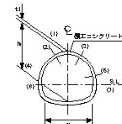
覆工コンクリート
