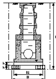
マンホール底部工
