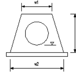
樋管工
