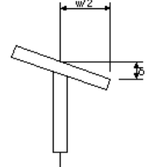
桁製作工(仮組立による検査を省略する 場合)(フランジの直角度)
