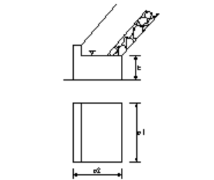
護岸基礎工_海岸コンクリートブロック工
