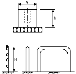
防止柵工(立入防止柵)(転落(横断)防止柵)(車止めポスト) 1
