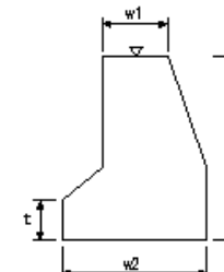
取付擁壁工(2)
