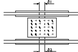
桁製作工(仮組立による検査を省略する 場合)(現場継手部のすき間)
