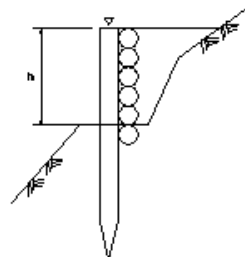
柵工
