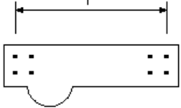
桁製作工(部材長)(プレートガーター)
