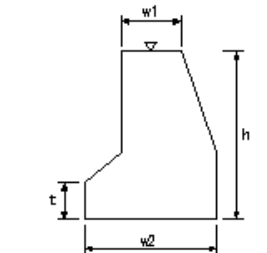
コンクリート擁壁工(2)
