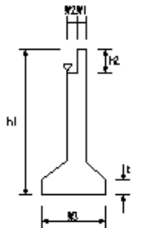
管理橋橋台工(3)
