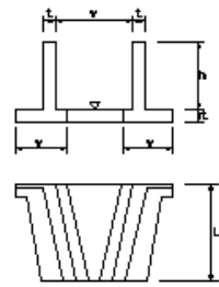
水叩工
