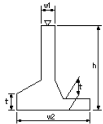
取付擁壁工(4)
