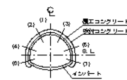
吹付工
