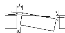
セルラー工(セルラー工据付)
