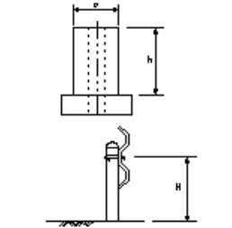
路側防護柵工(ガードレール)
