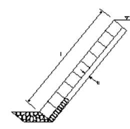
護岸工_海岸コンクリートブロック工
