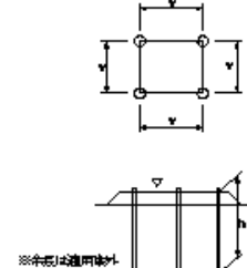
パーチカルドレーン工(サンドドレーン工)(ペーパードレーン工)(袋詰式サンドドレーン工)
