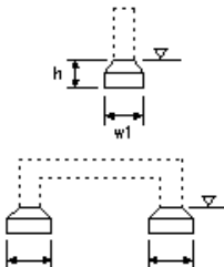
橋脚フーチング工(門型)1
