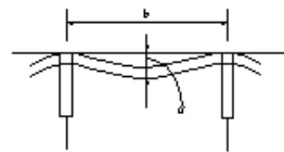
横断歩道橋製作工(板の平面度)
