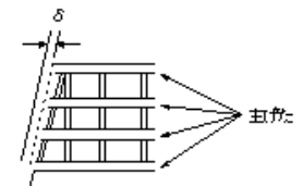
桁製作工(主桁、主構の橋端における出入り差)
