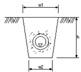
山腹暗渠工
