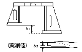
鋼製伸縮継手製作工(仮組立時)
