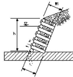
木製護岸工
