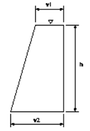
現場打擁壁工(1)
