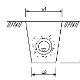
暗渠工(コルゲートパイプ)(ダクタイル鉄管)
