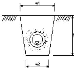
地下排水工
