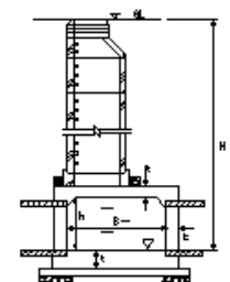
12/1/7/8現場打ち特殊人孔
