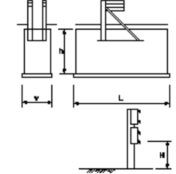
路側防護柵工(ガードケーブル)
