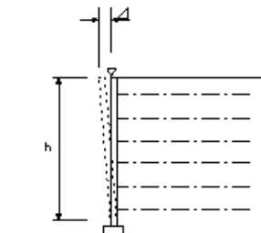
補強土壁工 補強土(テールアルメ)壁工 法、多数アンカー式補強土工法
