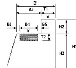
橋台各部
