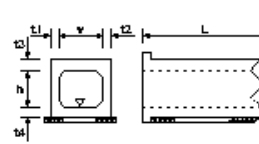
排水施設工(ボックスカルバート工・プレキャスト)
