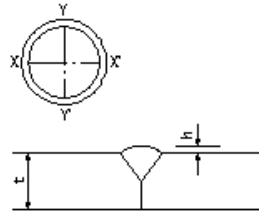
周継手溶接(余盛高)
