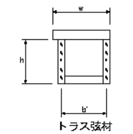
桁補強材製作工(トラス・アーチ等)
