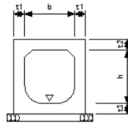
水路築造工(現場打水路)
