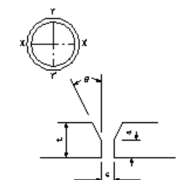
V型開先(片面溶接)
