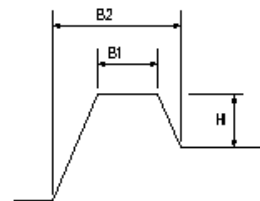
畦畔工
