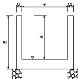
現場水路工
