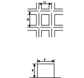
吹付枠工(梁間隔、梁断面)
