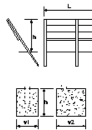
防雪柵工
