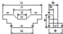
鋼製構造物(鋼製ダム)
