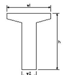
ポストテンションT(1)桁製作工
