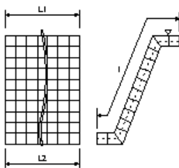
コンクリートブロック工(連結ブロック張り)
