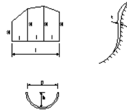
植生等の工種(伏工・吹付工類)
