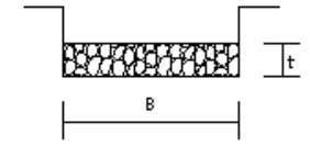
基礎工(置換基礎工・同木基礎工)
