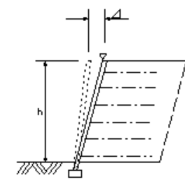
補強土壁工 ジオテキスタイルを用いた補強 土工法
