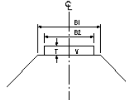
道路工(砂利道)
