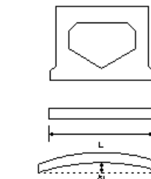
プレテンション桁購入工(スラブ橋)
