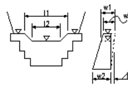
鋼製えん堤本體工(不透過型)
