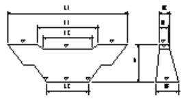
コンクリートダム (本ダム・副ダム)
