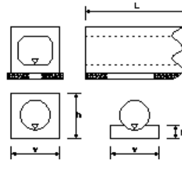
樋門接続暗渠工
