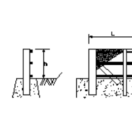
落石防護柵工
