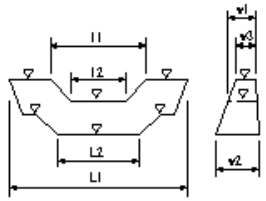
コンクリートえん堤本體工 コンクリート副えん堤工
