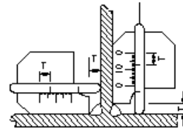
すみ肉溶接(脚長)
