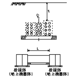
管路工
