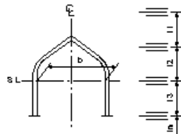
水路トンネル(支保工)
