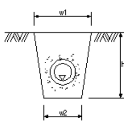
地下排水工
