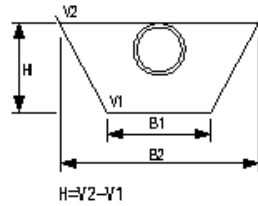
管水路基礎(砂基礎等)2
