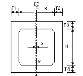
サイホン(現場打)
