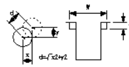
集水井工
