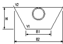
管水路基礎(砂基礎等)1
