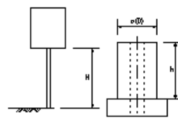
小型標識工
