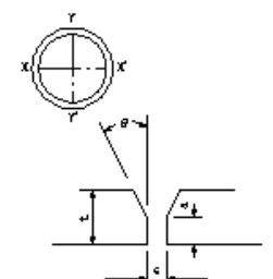
V型開先(両面溶接)
