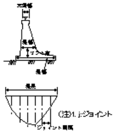
コンクリートダム工(本体)
