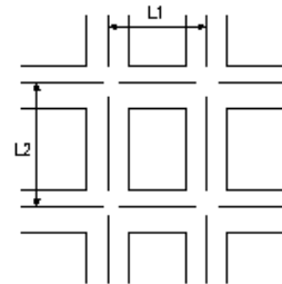
吹付枠工(梁間隔)
