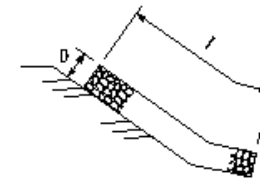
法面工(鉄線かご・かご擁壁・簡易鋼製土留擁壁)4
