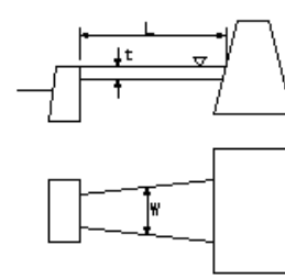
床固め工/水叩工
