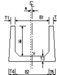
洪水吐工
