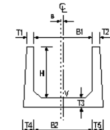
開水路(現場打)
