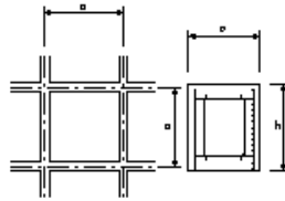
法枠工(現場打設工)(現場吹付法枠工)
