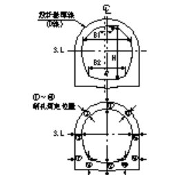
水路トンネル(コンクリート覆工)
