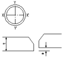
周継手溶接(目違い)
