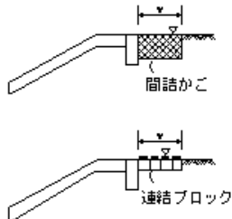
コンクリートブロック工(玉端保護ブロック)
