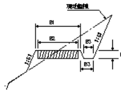
テラス(階段畑)
