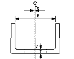
幅(B)、高さ(H)はL形水路のみ測定する
