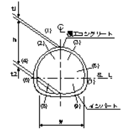
インパート本体工
