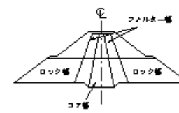
コアの盛立、フィルターの盛立、ロックの盛立
