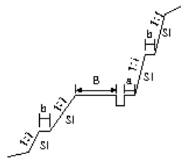
土工(切土・土取場・盛土・残土処理場)
