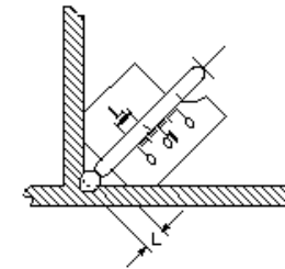
すみ肉溶接(のど厚)
