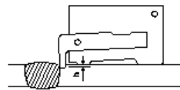
周継手溶接(アンダカット)
