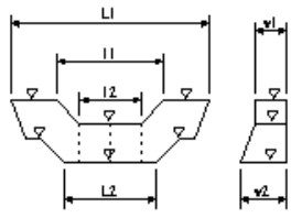
本堤工
