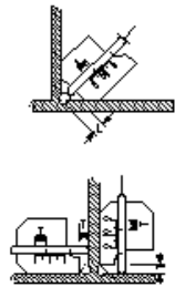
すみ肉溶接(脚長・のど厚)
