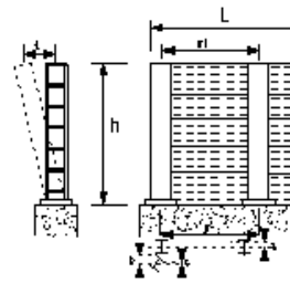
遮音壁本体工
