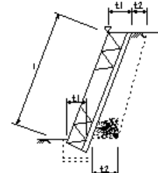
石積(張)工
