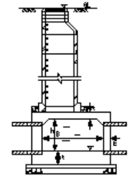
現場打ち特殊人孔
