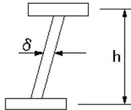
横断歩道橋製作工(仮組立による検査を省略する場合)(主桁、主構の鉛直度)
