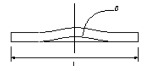
桁補強材製作工(圧縮材の曲がり)
