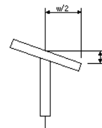
プレビーム用桁製作工(プレートガーター) プレビーム用桁製作工(フランジの直角度)
