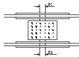
横断歩道橋製作工(仮組立による検査を省略する場合)(現場継手部のすき間)
