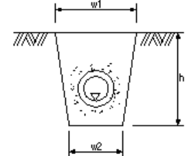
山腹暗渠工
