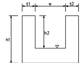
魚道工
