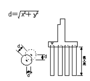
場所打杭工
