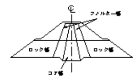
フィルターの盛立
