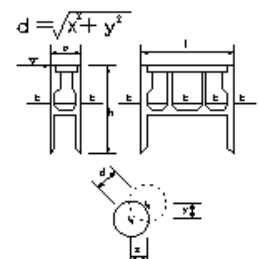
ニューマチックケーソン基礎工
