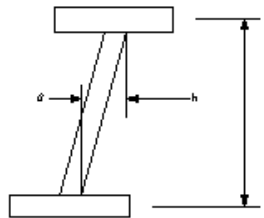
架設工(鋼橋)主げた、主構の鉛直度
