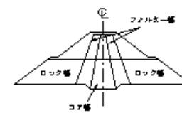
コアの盛立
