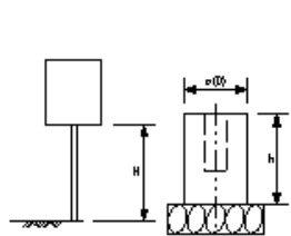
小型標識工
