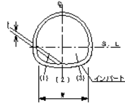
インパート本体工
