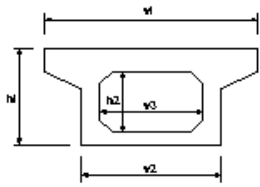
PC押し箱桁製作工
