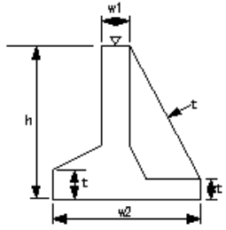
場所打擁壁工5
