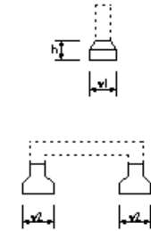
橋脚フーチング工(門型)
