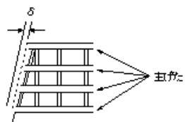
横断歩道橋製作工(仮組立による検査を省略する場合)(主桁、主構の橋端における廻り)
