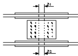
架設工(鋼橋)現場継手部のすき間
