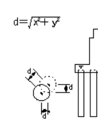
既製杭工(既製コンクリート杭)(鋼管杭)(H鋼杭)
