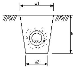
暗渠工
