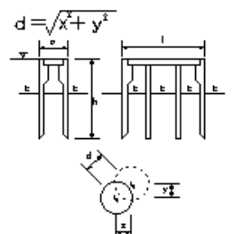
オープンケーソン基礎工
