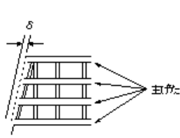
桁製作工(主桁、主構の橋端における出入り差)
