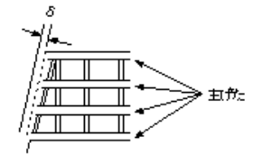
架設工(鋼橋)主げたの橋端における出入差
