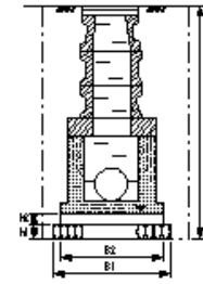
マンホール基礎工
