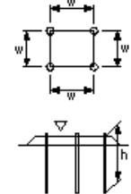
バッチカルドレーン工(サンドドレーン工)(ペーパードレーン工)(袋詰式サンドドレーン工)
