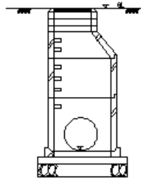
組立マンホール工
