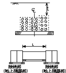
管路工
