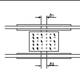
桁製作工(仮組立による検査を省略する場合)(現場継手部のすき間)
