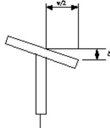
プレビーム用桁製作工(ワラジの直角度)
