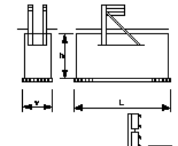
路側防護柵工(ガードケープル)
