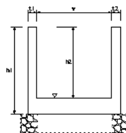
堤脚水路工
