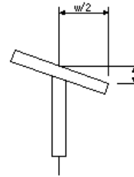
鋼桁補強工(フランジの直角度)
