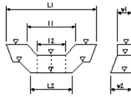
本堤工
