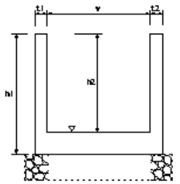
側溝工
