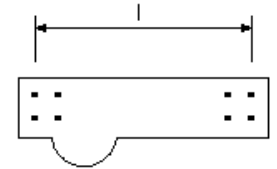
横断歩道橋製作工(仮組立による検査を省略する場合)(部材長)(プレートガーダー)
