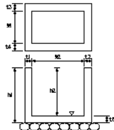
排水構造物修繕工(集水樹工)
