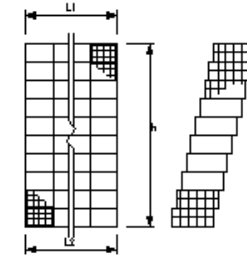
羽口工(ふとんかご)(かご枠工)
