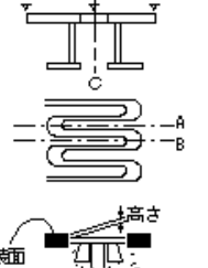
伸縮装置工(鋼フィンガージョイント)
