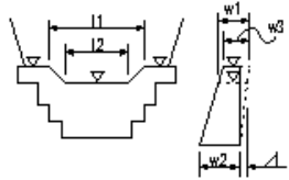
鋼製ダム本體工(不透過型)
