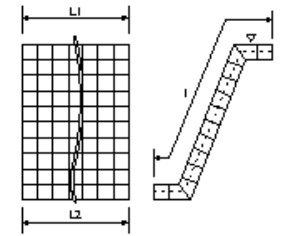
羽口工(連節ブロック張り工)
