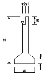
管理橋橋台工(3)
