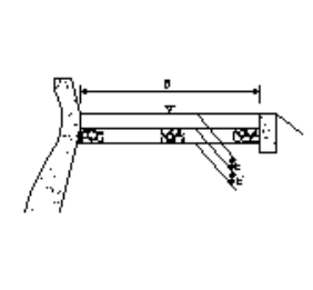
天端被覆工_コンクリート被覆工
