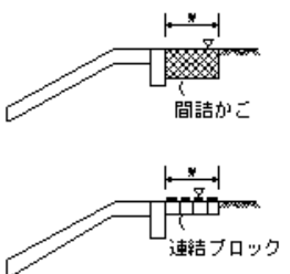
天端保護ブロック
