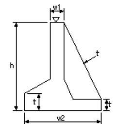
コンクリート擁壁工(5)
