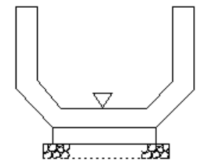
側溝工(プレキャストU型側溝)
