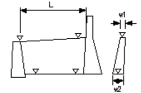
鋼製ダム工_コンクリート側壁工
