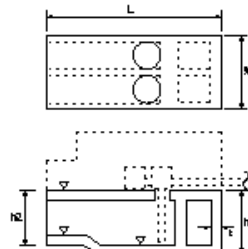
吐出水槽工(本体工)
