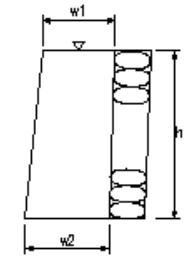
コンクリート擁壁工(3)
