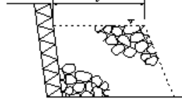
捨石工
