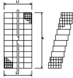
ふとんかご
