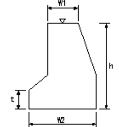
取付擁壁工(2)
