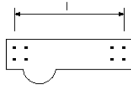
桁製作工(部材長)(プレートガーダー)
