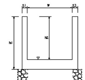
堤脚水路工
