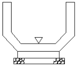
付帯道路工_プレキャストU型側溝
