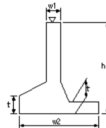
取付擁壁工(4)
