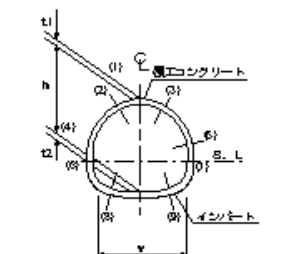
覆工コンクリート・側壁コンクリート
