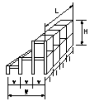
図a 格子形鋼製砂防ダム 鋼製ダム本體工(透過型)(図a)
