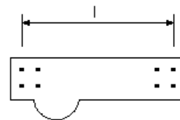
横断歩道橋製作工(部材長) (プレートガーター)
