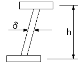
桁製作工(主桁、主構の鉛直度)
