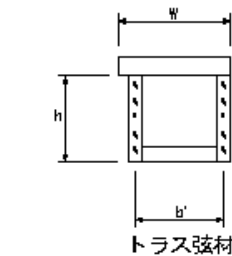
トラス弦材
