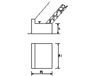
護岸基礎工_海岸コンクリートブロック工
