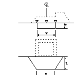
置換工
