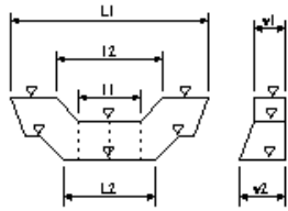
本堤工
