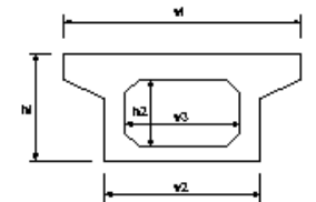
PC箱桁製作工
