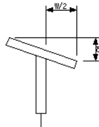
桁製作工(仮組立検査省略)クランジの直角度
