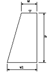
取付擁壁工(1)
