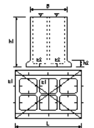
海城堤本体工_ケーソン工製作
