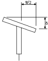
桁製作工(フランジの直角度)
