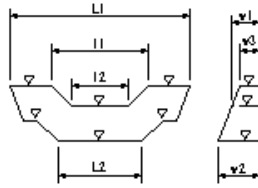
床固め本體工
