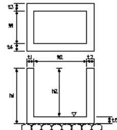
ハンドホール
