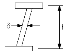
桁製作工(仮組立検査省略)主桁、主構の鉛直度
