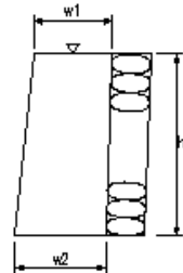
取付擁壁工(3)
