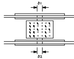
桁製作工(仮組立検査省略)(現場継手部のすき間)
