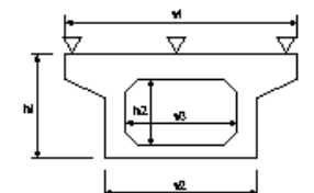
PC箱桁製作工・PC片持箱桁製作工
