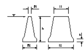
RC躯体工(重力式)(半重力式)
