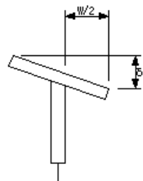
桁製作工(ワランジの直角度)
