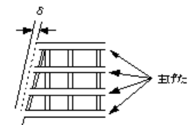
桁製作工(仮組立検査省略)(主桁、主構の橋端における出入差)
