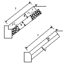
裏法被覆工_アスファルト被覆工
