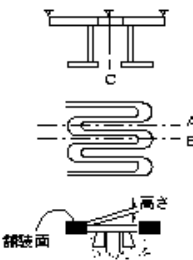
コンクリート管理橋上部工(鋼製フィンガージョイント)
