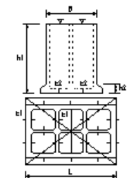
ケーソン工製作
