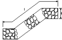
ジャカゴ工・かごマット工
