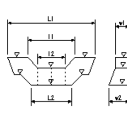
床固め本体工
