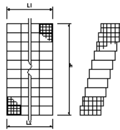
ふとんかご
