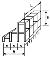
図a 格子形鋼製砂防ダム 鋼製ダム製作工(仮組立時)(図a)
