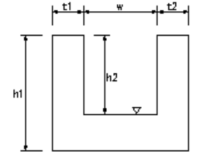
魚道工
