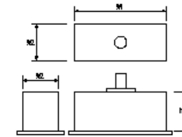
標識基礎工
