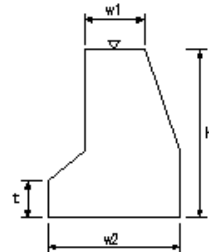
取付擁壁工(2)
