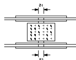
桁製作工(現場継手部のすき間)
