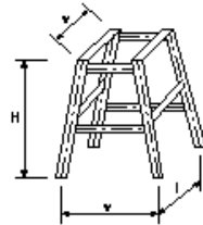
図c 鋼製スリットダムB型 鋼製ダム製作工(仮組立時)(図c)
