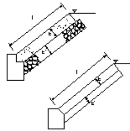
裏法被覆工_コンクリート被覆工
