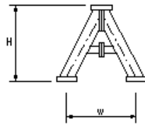
図b 鋼製スリットダムA型 鋼製ダム本體工(透過型)(図b)
