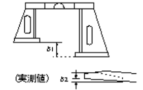
工場製作工_鋼製伸縮継手製作工(仮組立時)
