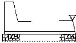
付帯道路工_L型側溝
