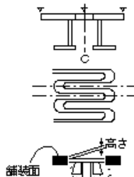
橋梁付属物工_伸縮装置工(鋼フィンガージョイント)
