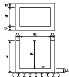
集水桝工
