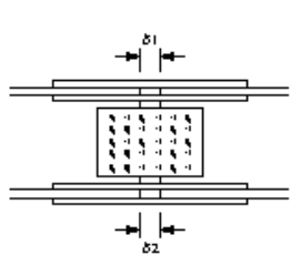
桁製作工(仮組立検査省略)(現場継手部のすき間)
