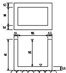
集水桝・マンホール工
