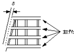
桁製作工(仮組立検査省略)(主桁、主構の橋端における出入差)
