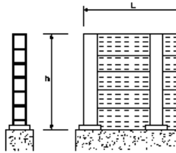
遮音壁本体工
