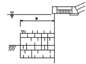
沈床工
