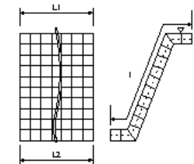
連節ブロック張り
