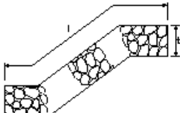
じゃかご
