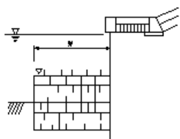
水制工_沈床工
