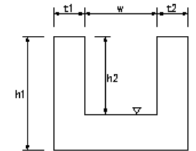
魚道本体工
