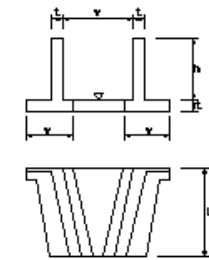
翼壁工
