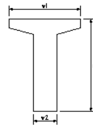
ポストテンションT(D)桁製作工
