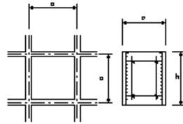
矢板工(指定仮設・任意仮設は除く)(鋼矢板)(軽量鋼矢板)(コンクリート矢板)...
