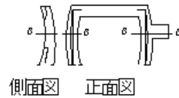
鋼製橋脚製作工(仮組立時)(おのきアンバー及び柱の曲がり)
