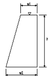
小型擁壁工
