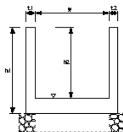
堤脚水路工
