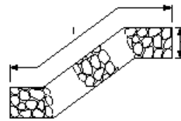
羽口工(じゃかご)
