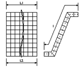
連節ブロック張り工
