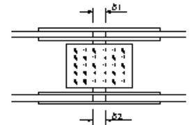
横断歩道橋製作工(現場継手部のすき間)
