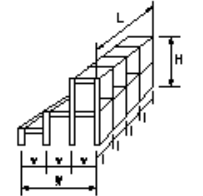
図a 格子形鋼製砂防ダム
