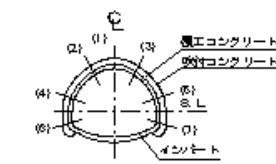
吹付工
