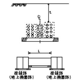
管路工
