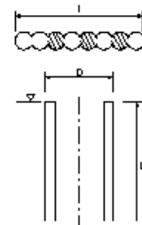
地中連続壁工(柱列式)
