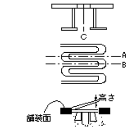
伸縮装置工(鋼フィンガージョイント)
