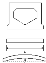
プレテンション桁梁工(スラブ桁)
