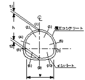
インパート本体工
