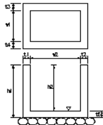
集水枳工
