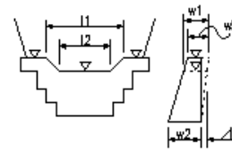
鋼製えん堤本体内工(不透過型)
