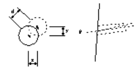
集排水ボーリング工 d = \sqrt{R^2 + Y^2}
