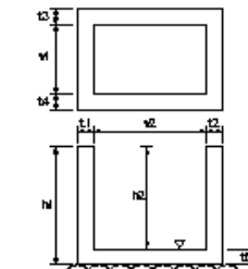
集水樹工
