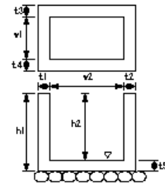
集水樹工
