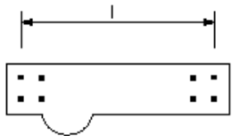
桁製作工 部材長(鋼けた)
