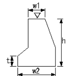
場所打擁壁工(2)
