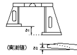
鋼製伸縮継手製作工(仮組立時)
