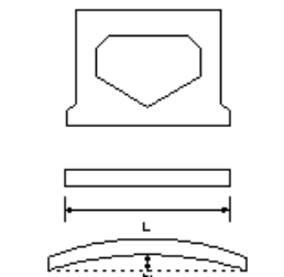
プレキャスト用桁購入工(スラブ橋)
