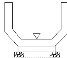
プレキャストカルバート工(プレキャストブロック工) プレキャストカルバート工(プレキャストパイプ工) 側溝工(プレキャストU型側溝工) (コリゲート) (フリーム) (自由勾配側溝)
