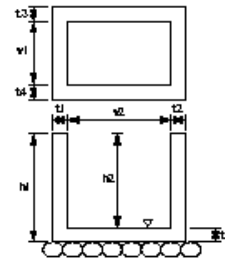
集水樹工
