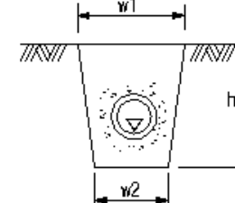
暗渠工
