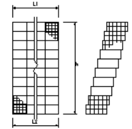
かご工(ふとんかご)
