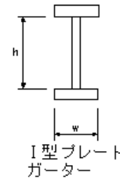
プレーム用桁製作工(プレートガーター)
