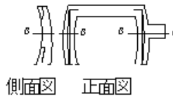
鋼製橋脚製作工(仮組立時)(はりのキャムバー及び柱の曲がり)
