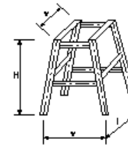
図c 鋼製スリットダムB型 鋼製ダム本體工(透過型)(図c)
