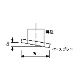
鋼製橋脚製作工 部材(脚柱とベースプレートの鉛直度)
