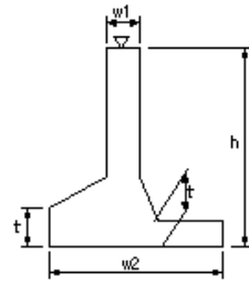
コンクリート擁壁工(4)
