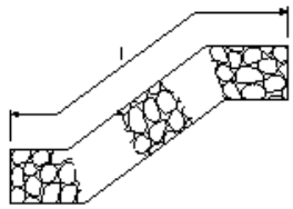
かご工(じゃかご)
