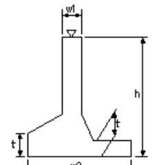
取付擁壁工(4)
