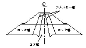
ロックの盛立
