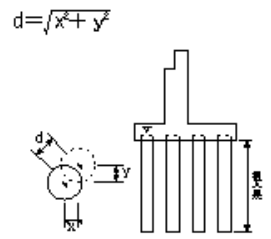
既製杭工
