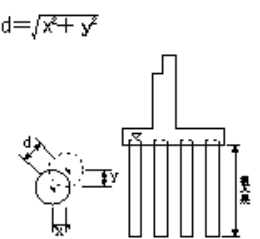
場所打杭工
