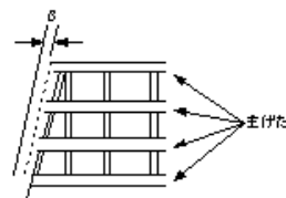
桁製作工(主けた、主構の橋端における出入差)
