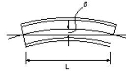
桁製作工(主桁、主構のそり)
