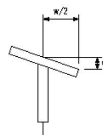
プレキャストカルバート工(フランジの直角度)
