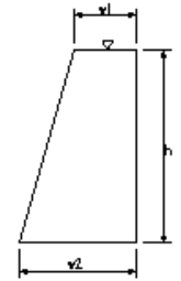
現場打擁壁工(1)
