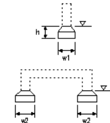
橋脚フーチング工(門型)
