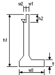
橋台躯体工(4)
