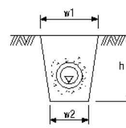
暗渠工
