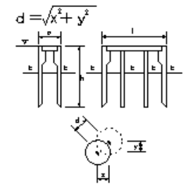
オープンケーソン基礎工
