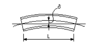
プレキャストカルバート工 仮組立時 主筋のそり
