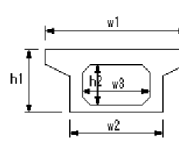
PC押し出し箱桁製作工
