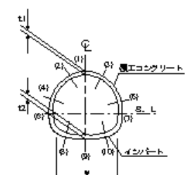
インパート本体工 1
