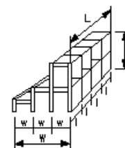
図a 格子形鋼製砂防ダム 鋼製堰堤本體工(透過型)(図a)
