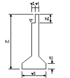
アンカーフレーム製作工
