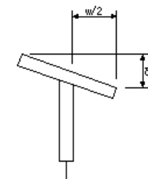
プレーム用桁製作工(フランジの直角度)
