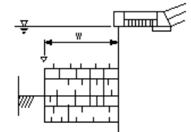
沈床工
