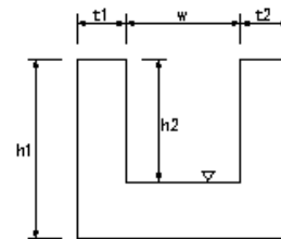
側溝工
