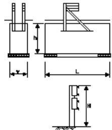
路側防護柵工(ガードケーブル)
