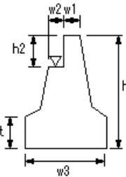
橋台躯体工(1)
