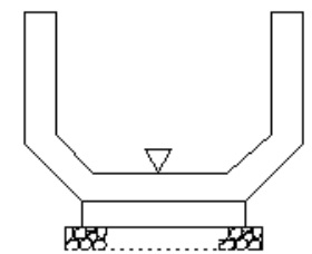
側溝工_プレキャストU型側溝・自由勾配側溝
