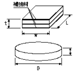
casting 工(大型ゴム支承工)
