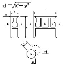
ニューマチックケーソン基礎工
