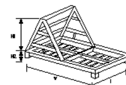
図d 鋼製L型スリットダム 鋼製堰堤本體工(透過型)(図d)
