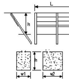
防雪柵工
