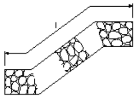
縁切工(じゃかご工)
