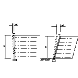
補強土壁工
