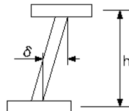
桁製作工(主けた、主構の鉛直度)
