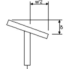
プレキャスト用桁製作工(フランジの直角度)
