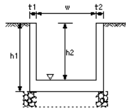
現場水路工
