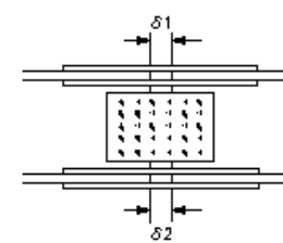
桁製作工(現場継手部のすき間)
