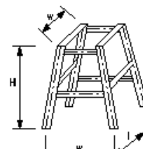
図c 鋼製スリットダムB型 鋼製堰堤本體工(透過型)(図c)
