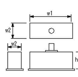
大型標識工(標識基礎工)
