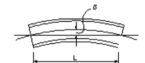
桁製作工(主桁、主構のそり)
