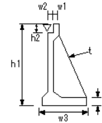
橋台躯体工(2)
