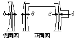
鋼製橋脚製作工(仮組立時)(柱のセンター間隔及び柱の曲がり)
