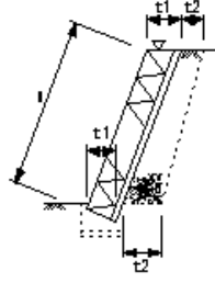
石積(長)工
