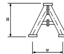
図b 鋼製スリットダムA型 鋼製ダム本体工(透過型)(図b)
