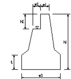
橋台躯体工(1)
