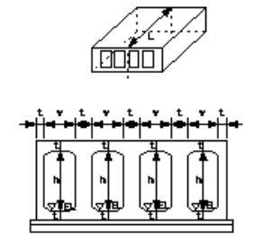
現場打ちボックス工(特殊部)
