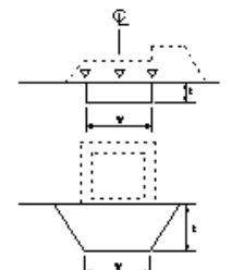
置換工
