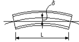
プレーム用桁製作工 仮組立時 主桁のそり
