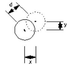
d = \sqrt{x^2 + y^2} 土留・仮締切工(アンカー工)
