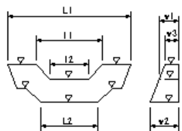
コンクリートダム本体工
