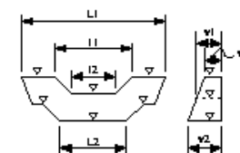
本体工(床固め本体工)
