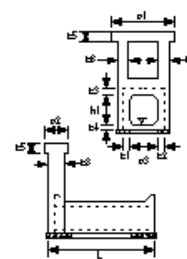
函渠工(本体工)
