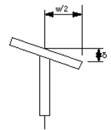
桁補強材製作工(フランジの直角度)
