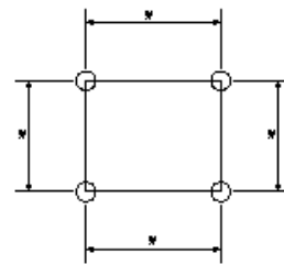
パチカルドレーン工(サンドドレーン工)(ベ ーパドレーン工)(袋詰式サンドドレーン工) 固結工(粉体噴射攪拌工)(高圧噴射攪 拌工)(スラリー攪拌工)(生石灰パイル工)
