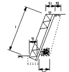
石積(長)工
