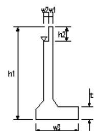
橋台躯体工(4)
