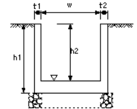
現場打水路工
