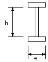
I型鋼ぎた プレビュー用製作工(フランジ幅、腹板高)
