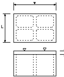
ケーソン工(突堤上部工)/場所打ちコンクリート_海岸コンクリートブロック
