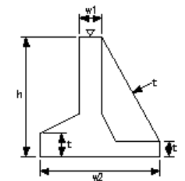
場所打擁壁工(5)
