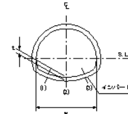
インパート本体工
