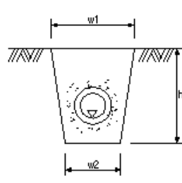
地下排水工
