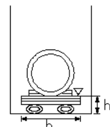
はしご胴木基礎
