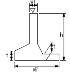
場所打擁壁工(4)
