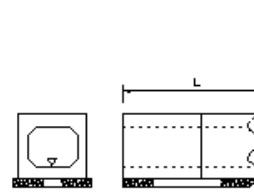
インパート本体工
