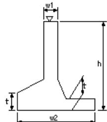
コンクリート擁壁工(4)
