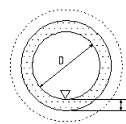
二次覆工
