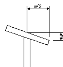
桁製作工(フランジの直角度)
