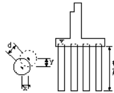
深礎工
