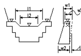
鋼製ダム本体工(不透過型)
