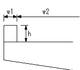
地覆工
