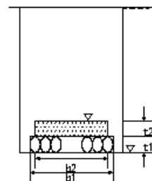
立坑土工
