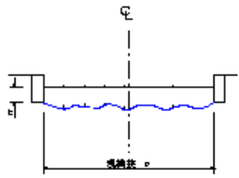
路上表層再生工
