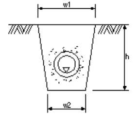
暗渠工
