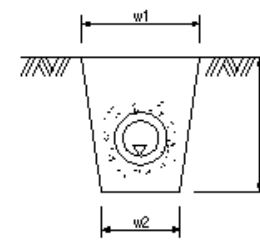
暗渠工(コルゲートパイプ)(ダクタイル铸铁管)
