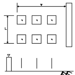
杭出し水制工
