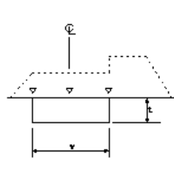
路床安定処理工 1
