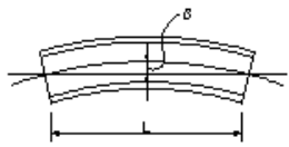
横断歩道橋製作工(主桁、主構のそり)
