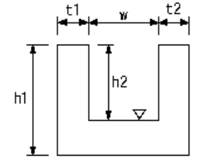
魚道工 1 1
