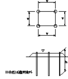
バッチカルドレーン工(サンドドレーン工) (バ →バードレーン工) (袋詰式サンドドレーン 固結工(粉体噴射攪拌工) (高圧噴射攪 拌工) (セメントミルク攪拌工) (生石灰バ...
