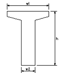
ポストテンションT(1)桁製作工
