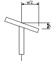
鋼桁補強工(フランジの直角度)
