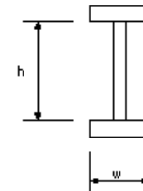
I型プレートガーター
