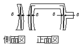
鋼製橋脚製作工(仮組立時)(はりのキャンバー及び柱の曲がり) 鋼製橋脚製作工(仮組立時)(柱の鉛直度)
