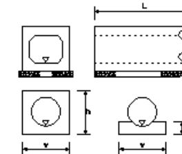
プレキャストカルバート工
