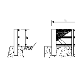
落石防護柵工
