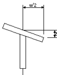
部材 プレキャスト用桁製作工(フランジの直角度)
