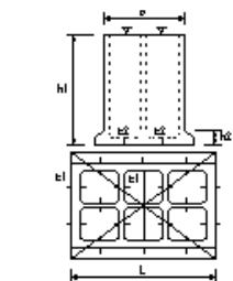
ケーソン工(ケーソン工製作)
