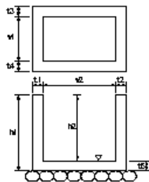
集水桝・マンホール工
