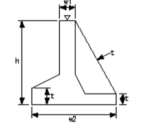
場所打擁壁工(5)
