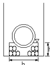
碎石基礎
