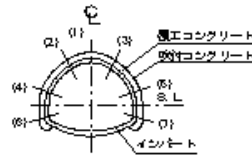
吹付工
