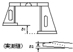
鋼製伸縮継手製作工(板組立時)
