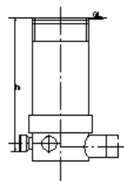
公共ます
