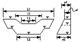
コンクリート堰堤本体工
