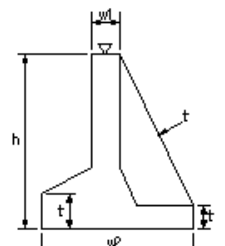
取付擁壁工(5)
