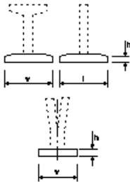
橋脚フーチング工(Ⅰ型)(T型)
