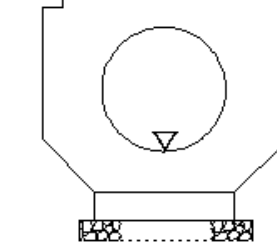
側溝工(管(函)渠型側溝工)管渠工
