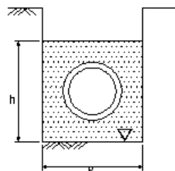
砂基礎
