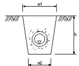
地下排水工
