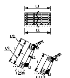
井桁ブロック工
