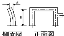
鋼製橋脚製作工(仮組立時)(はりのキャンバー及び柱の曲がり) 鋼製橋脚製作工(仮組立時)(柱の鉛直度)
