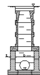
標準マンホール工
