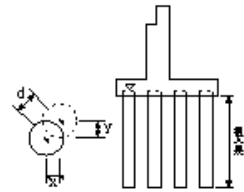
場所打杭工
