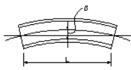
プレビーム用桁製作工(仮組立時 主桁のそり)
