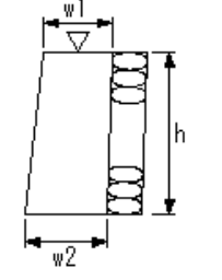
場所打擁壁工(3)
