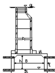
現場打ち特殊人孔
