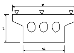
PCホロースラブ製作工・RC場所打ホロースラブ製作工・PC版桁製作工
