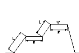
盛土・切土
