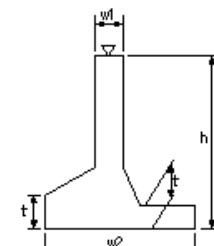
取付擁壁工(4)
