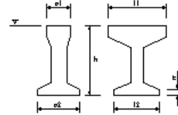
RC躯体工(張出式)
