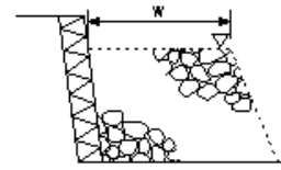
捨石工
