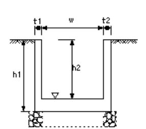
現場排水路工
