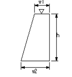
場所打擁壁工(1)
