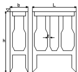
ケーソン基礎
