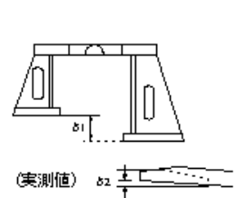
鋼製伸縮継手製作工(仮組立時)
