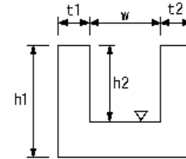
魚道工 1
