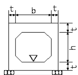
現場打水路
