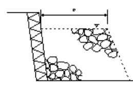
捨石工
