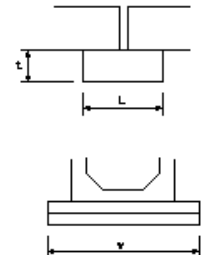
カラー継手工
