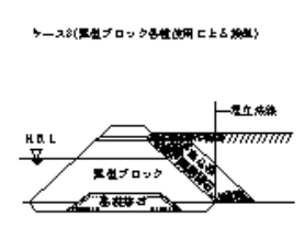
埋立てケース8(異型ブロック各種使用による護岸)
