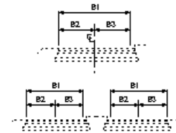
アスファルト・半たわみ性・排水性・グースアスファルト・コンクリート舗装工(表層工)
