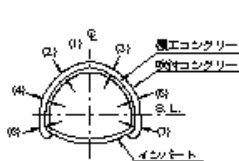
吹付けコンクリート
