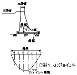
コンクリートダム工(本体)
