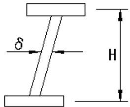
横断歩道橋製作工(主げたの鉛直度)
