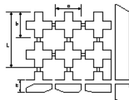
護岸基礎工(海岸コンクリートブロック工)
