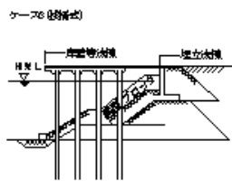
埋立てケース6(桁橋式)
