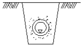
地下排水工(暗渠工)(樋門接続暗渠工)
