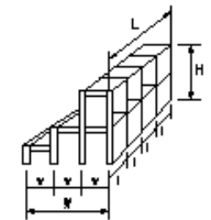
図a 格子形鋼製砂防ダム 砂防鋼製ダム本体内工(透過型)(図a)
