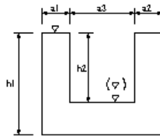
側溝(▽)水路 山腹U型側溝工
