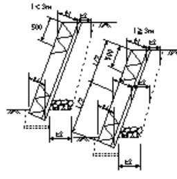
コンクリートブロック積工・コンクリートブロック張工・緑化ブロック工・石積(長)工
