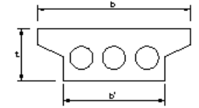
PCホロースラブ製作工・RC場所打・木口スラブ製作工・PC版桁製作工
