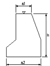
現場打擁壁工(2)
