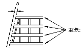
横断歩道橋製作工(主げたの橋端における出入り差)
