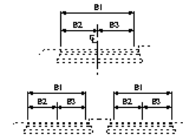
アスファルト・半たわみ性・排水性・グースアスファルト・コンクリート舗装工(下層路盤工)
