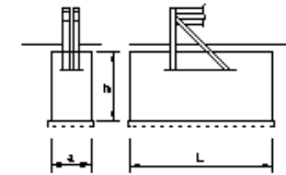
路側防護柵工(ガードケーブル)コンクリートケーブル取付け
