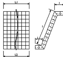
連節ブロック工・かごマット工(標準タイプ)
