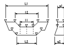
砂防床固め本体内工・垂直壁工
