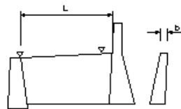
砂防コンクリート側壁工
