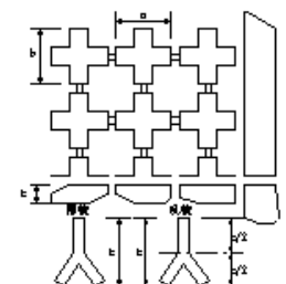
根固め工・消波ブロック工(根固めブロック工)・消波ブロック工
