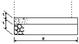
基礎材(栗石・クラッシャーラン)均しコンクリート
