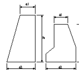
護岸工(直立掘)
