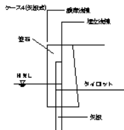
埋立てケース4(矢板式)
