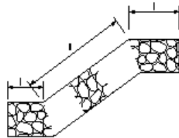
蛇籠部長工
