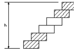
布団籠工・かごマット工
