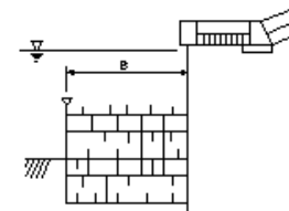
沈床工 そだ沈床・木工沈床・改良沈床
