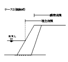
埋立てケース2(傾斜式)
