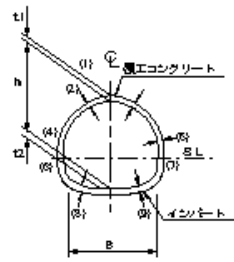
トンネル(覆工)
