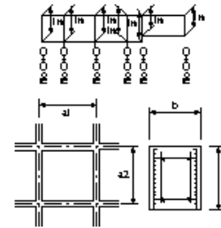
現場打法枠工・現場吹付法枠工(1)
