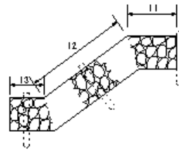
蛇籠長工
