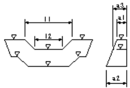
砂防コンクリートダム本体内工副堰堤
