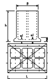
突堤本体工(ケーソン工製作)
