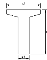
ポストテンションT(⊥)桁製作工
