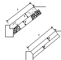
護岸工(コンクリート被覆工)・天端被覆工(アスファルト、コンクリート被覆工)・裏法
