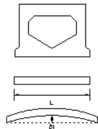
プレテンション桁工(スラブ橋)
