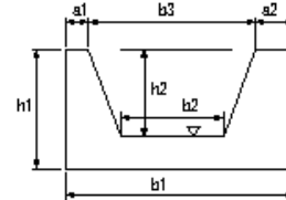
コンクリート三面張流路工
