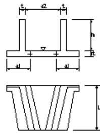
翼壁工及び水叩工
