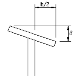
桁製作工(フランジの直角度)
