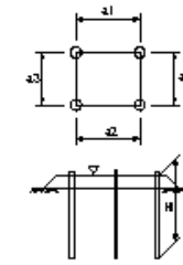
パーティカルドレーン工(サンドドレーン工、ペーパードレーン工、袋詰式サンドドレーン工)
