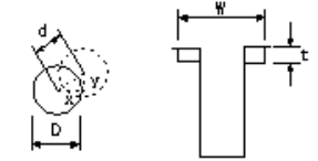
集水井工
