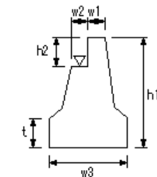
橋台躯体工(1)
