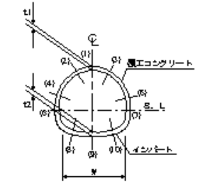
インパート本体工
