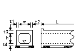
場所打函渠工
