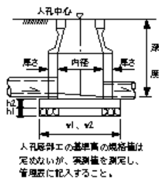
下水道用人孔
