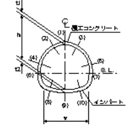
覆工コンクリート・側壁コンクリート
