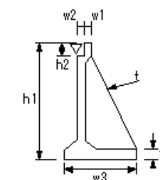
橋台躯体工(2)
