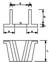
翼壁工・水叩工
