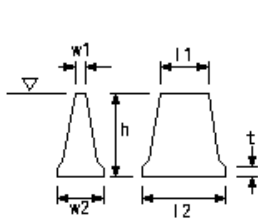
RC躯体工(重力式)(半重力式)
