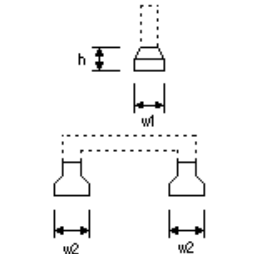
橋脚フーチング工(門型)
