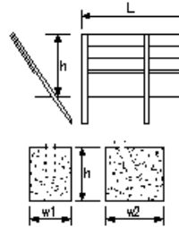
防雪柵工
