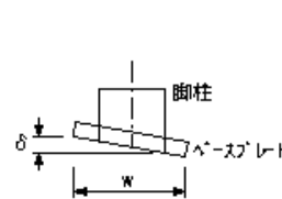
鋼製橋脚製作工(部材)(脚柱とベースプレートの鉛直度)
