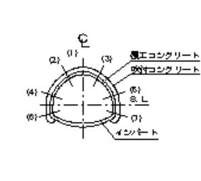
吹付工
