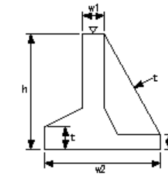
場所打擁壁工(5)
