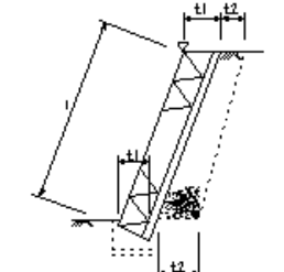
石積(石)工
