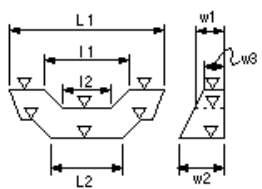
本體工(床固め本體工)
