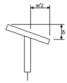
プレキャスト用桁製作工(フランジの直角度)
