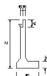
管理橋橋台工(4)
