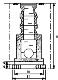
マンホール基礎工
