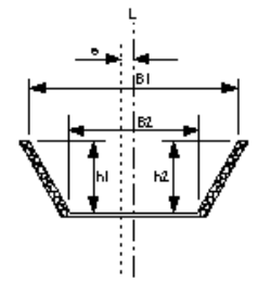
ライニング水路(コンクリート二次製品)
