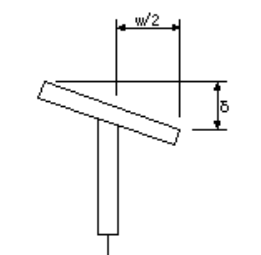
プレビーム用桁製作工(フランジの直角度)
