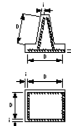
鉄筋の組立て
