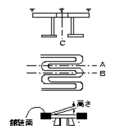
橋梁付属物工_鋼製フィンガージョイント
