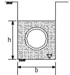
砂基礎
