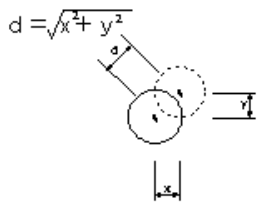
既製杭工
