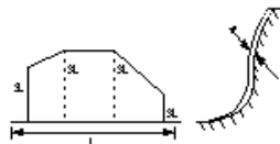
吹付工
