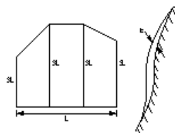
植生工_植生基材吹付工
