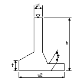
可動堰本体工_取付擁壁工(4)
