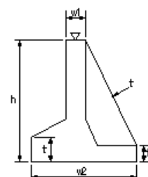
固定堰本体工_取付擁壁工(5)
