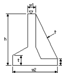
擁壁工(5)
