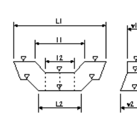
本体工(床固め本体工)
