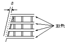
桁製作工(主桁、主構の橋端における出入差)
