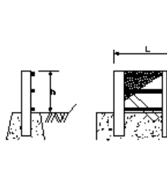
落石防護柵工
