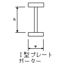
プレビーム用桁製作工(プレートガーター)
