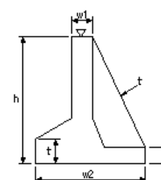
現場打擁壁工(5)
