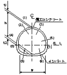
インパート本体工
