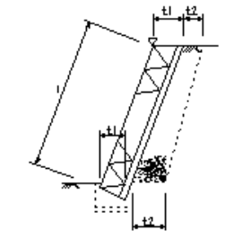
石積(張)工
