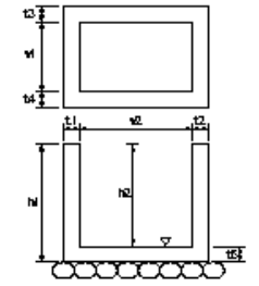
排水構造物修繕工(集水栞工)
