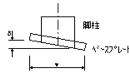
鋼製橋脚製作工(部材)(脚柱とベースプレートの鉛直度)
