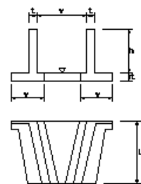
翼壁工
