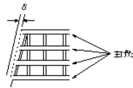
架設工(主桁、主構の橋端における出入差)
