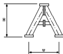
図b 鋼製スリットダムA型 鋼製ダム本体工(透過型)(図b)
