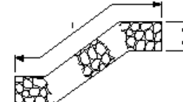
根固め工(かご工(じゃかご)(かごマット)
