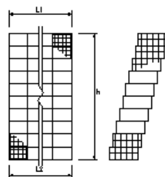
かご工(ふとんかご工)
