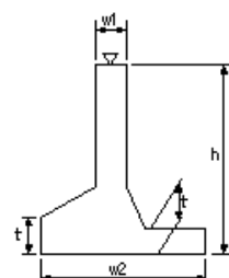
固定堰本体工_取付擁壁工(4)
