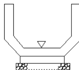
側溝工(プレキャストU型側溝)(自由勾配)
