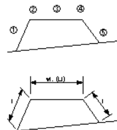
突堤本体工_捨石工
