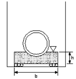
コンクリート基礎
