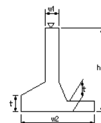
取付擁壁工(4)
