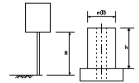
小型標識工
