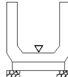
側溝工(プレキャストU型側溝)(コリゲート フリューム)(自由勾配側溝)
