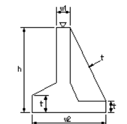
可動堰本体工_取付擁壁工(5)
