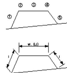
海城堤基礎工_捨石工
