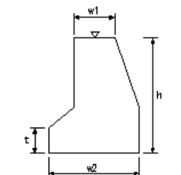
可動堰本体工_取付擁壁工(2)
