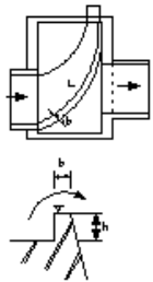
越流堰(雨水吐室)
