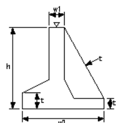
現場打擁壁工・土留工(5)
