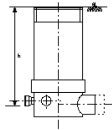
公共ます
