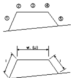
護岸基礎工_捨石工
