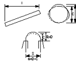
コルゲートパイプ工・合成樹脂管
