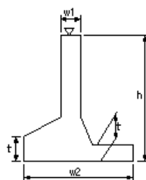
擁壁工(4)
