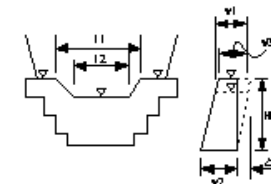
鋼製ダム本體工(不透過型)
