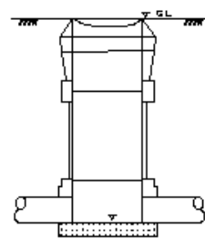
小型マンホール工
