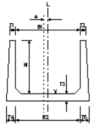
フリューム
