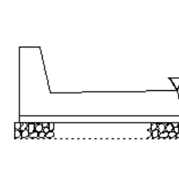
側溝工(L型側溝)
