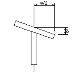
横断歩道橋製作工(フランジの直角度)
