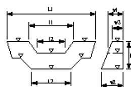
コンクリートダム工_床固工
