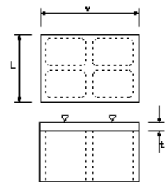
セルラー工(突堤上部工)/場所打コンクリート・海岸コンクリートブロック
