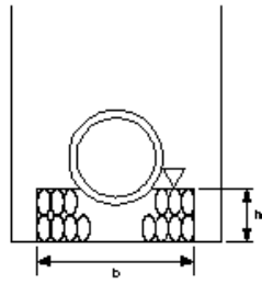
碎石基礎
