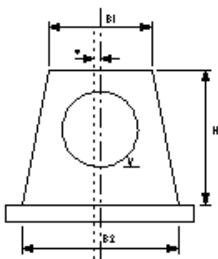
樋管工
