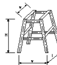
図c 鋼製スリットダムB型 鋼製ダム本体工(透過型)(図c)
