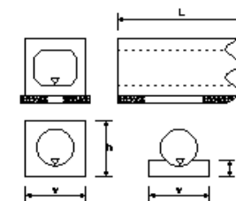
函渠工(PC函渠)
