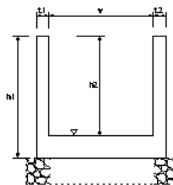
側溝工
