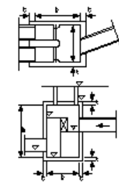
伏せ越し室・雨水吐室
