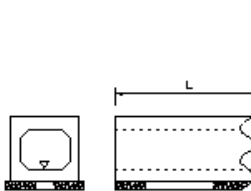
裏法被覆工_コンクリート被覆工
