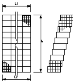
水制工(かご工(ふとんかご)
