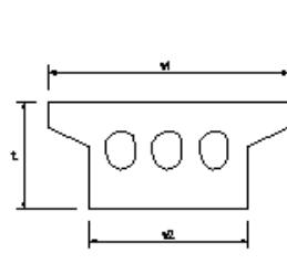
PCホロースラブ製作工
