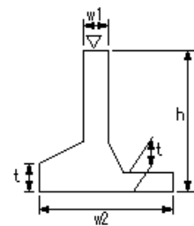
地下水遮断工_現場打擁壁工(4)
