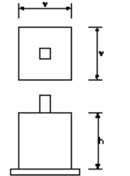
組立歩道工(支柱基礎工)
