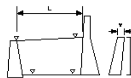
側壁工
