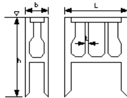
ケーソン基礎
