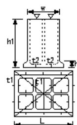
ケーソン工製作
