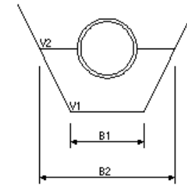
砂基礎
