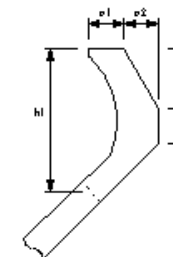
波返工
