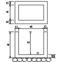
街渠樹・マンホール工(街渠樹工)(マンホール工)
