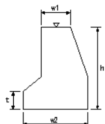
固定堰本体工_取付擁壁工(2)
