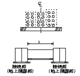
管路工(管路部)
