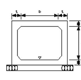
現場打水路
