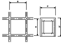
法枠工(現場打枠工)(現場吹付法枠工)
