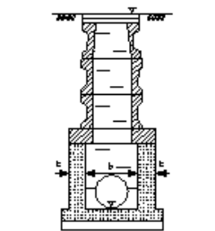
標準マンホール工
