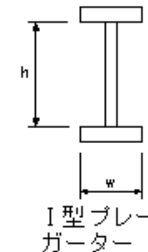
桁製作工(プレートガーター)
