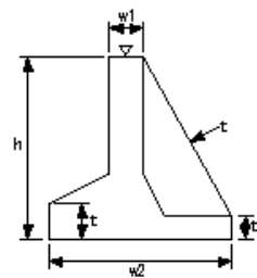
地下水遮断工_現場打擁壁工(5)
