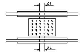
桁製作工(現場継手部のすき間)
