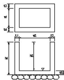
集水樹工
