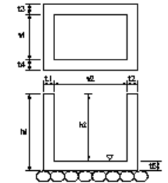
街渠樹・マンホール工(街渠構工)(マンホール工)
