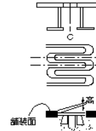
伸縮装置工(鋼フィンガージョイント)
