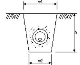
山腹暗渠工
