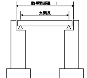
躯体工(5)
