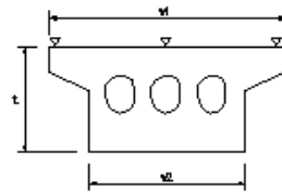
PC木口スラブ製作工
