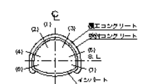
吹付工
