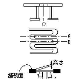
伸縮装置工(鋼フィンガージョイント)
