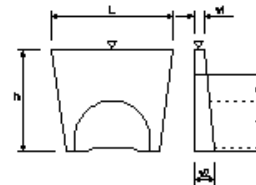
坑門本体工
