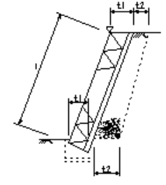
石積(張)工
