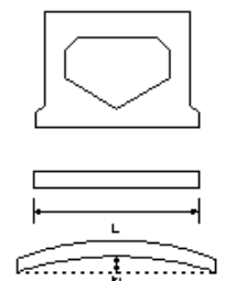
プレテンション桁購入工(スラブ桁)
