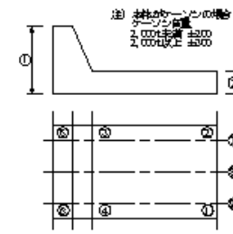
防波堤
