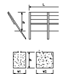
防雪柵工
