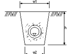
山腹暗渠工
