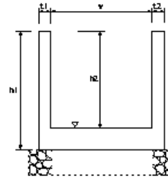
側溝工
