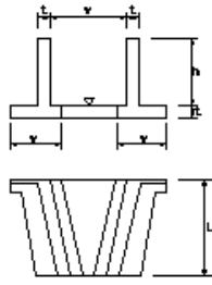
翼壁工
