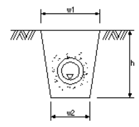
暗渠工
