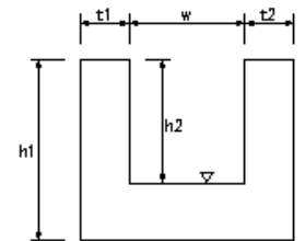
魚道本体工
