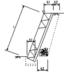
石積(張り)工
