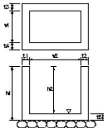
集水枳工
