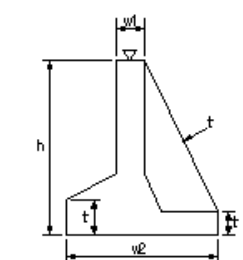
取付擁壁工(5)
