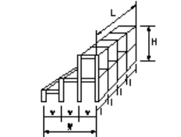
図a 格子形鋼製砂防ダム
