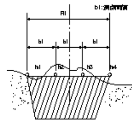
置換え
