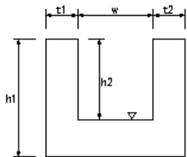
側溝工
