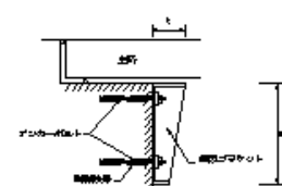
落橋防止工
