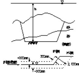
床掘
