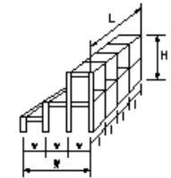
図a 格子形鋼製砂防ダム 鋼製ダム製作工(仮組立時)(図a)
