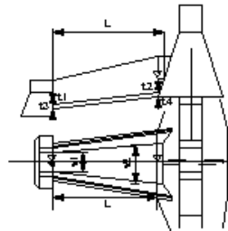
コンクリートダム工_水叩工
