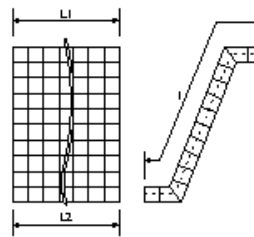
土留・仮締切工(連節ブロック張り工) 1)
