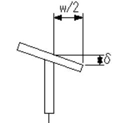
プレビーム用桁製作工(フランジの直角度)
