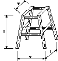
図c 鋼製スリットダムB型
