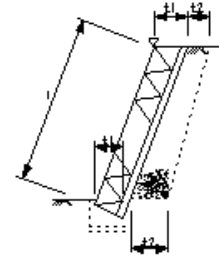
多自然型護岸工(巨石張り)巨石積み 多自然型護岸工(ふとんかご工)かごマット
