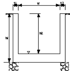
魚道本体工
