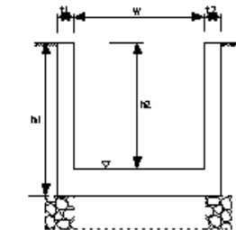
堤脚水路工
