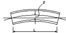
桁製作工(主桁、主構のそり)
