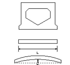
プレテンション桁購入工(スラブ橋)
