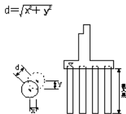
5 場所打杭工
