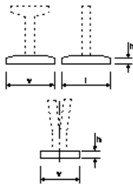
橋脚フーチング工 (直型) (T型)
