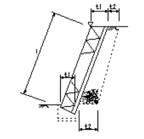
石積(長)工
