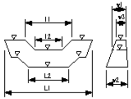
コンクリートダム本体工・コンクリート副ダム工・垂直壁工
