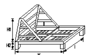
図d 鋼製L型スリットダム
