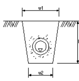
暗渠工(コルゲートパイプ)(ダクタイル鋳鉄管)
