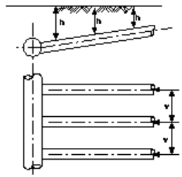
吸水渠工
