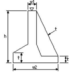
現場打擁壁工(5)
