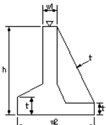
取付擁壁工(5)
