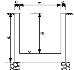
現場打水路工
