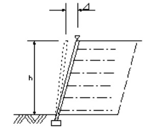
補強土壁工(ワイヤーウォール工法)
