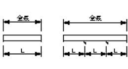
横断歩道橋製作工 (全長、支間長)
