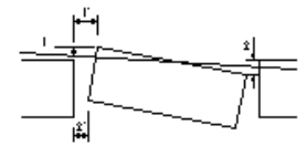
ケーソン工(ケーソン工据付)
