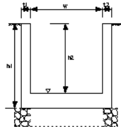
側溝工
