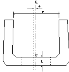
二次製品水路工(L型、大型フリューム)
