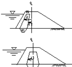
コアの盛立
