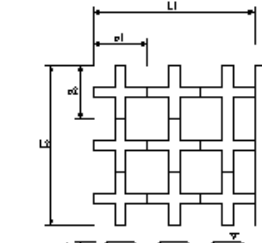
本体工(根固めブロック)
