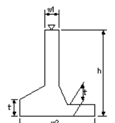
取付擁壁工(4)
