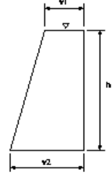
現場打擁壁工(1)
