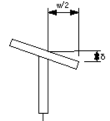
桁製作工(フランジの直角度)
