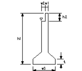
軀体工(3)
