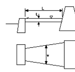
床固め工/水叩工
