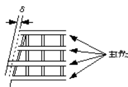
架設工(鋼橋)主けたの橋端における出入差(※仮組立検査省略)
