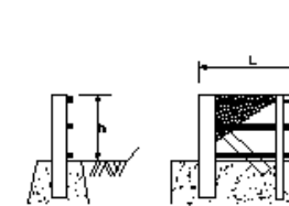
落石防護柵工
