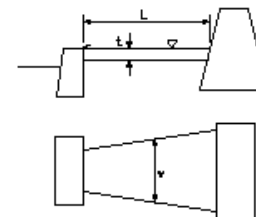
鋼製ダム工_水叩工
