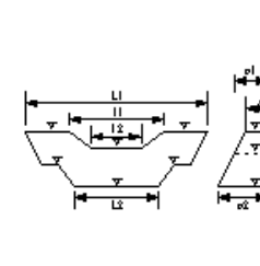
本体工(床固め本体工)
