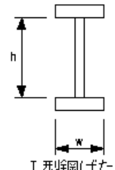
桁製作工(仮組立による検査を省略する場合)(鋼(げた))
