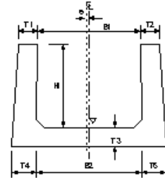
洪水吐工
