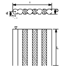
地中連続壁工(柱列式)
