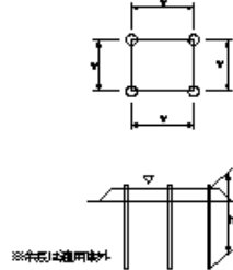
パーカドレーン工(サンドドレーン工)(ペーパードレーン工)(袋詰式サンドドレーン工)
