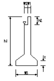
管理橋橋台工(3)
