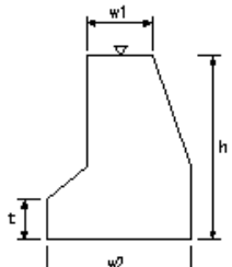
取付擁壁工(2)
