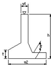
取付擁壁工(4)
