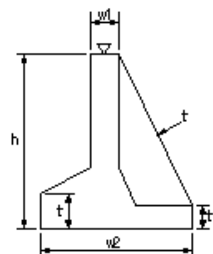
取付擁壁工(5)
