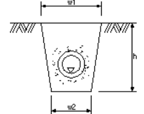
山腹暗渠工
