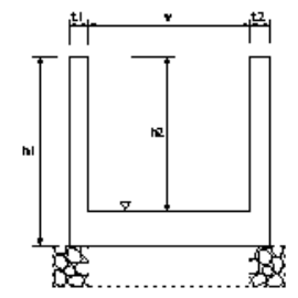
現場水路工
