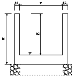
側溝工
