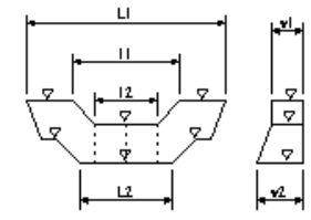
本堤工
