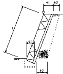
石積(長)工
