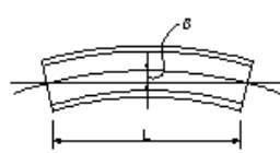
仮組立時 主桁のそり
