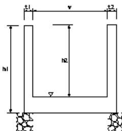
堤脚水路工
