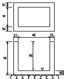
集水枡工
