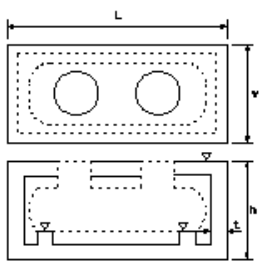
燃料貯油槽工
