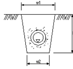
暗渠工
