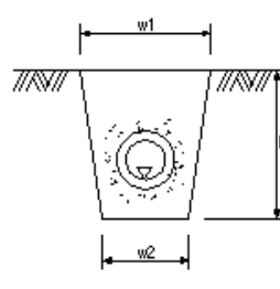
地下排水工
