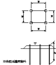
パチカルドレーン工(サンドドレーン工) (ペーパードレーン工)(袋詰式サンドドレーン工) ※布材は適用除外
