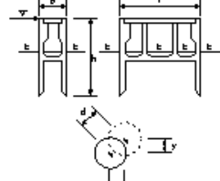
ニューマチックケーソン基礎工
