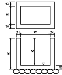
街渠溝・マンホール工(街渠樹工)(マンホール工)
