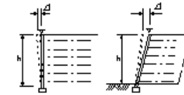
補強土壁工
