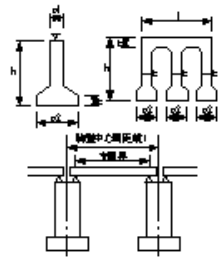
RC躯体工(ラーメン式)
