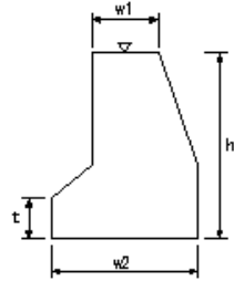
取付擁壁工(2)
