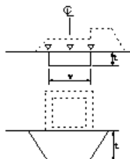
置換工
