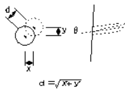
アンカー工 d = \sqrt{x^2 + y^2}
