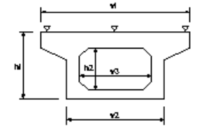
PC桁筋製作工
