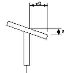
鋼桁補強工(フランジの直角度)
