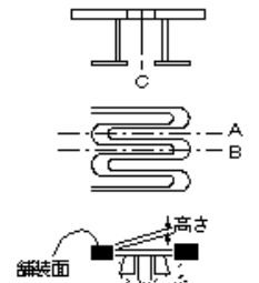
橋梁付属物工(伸縮装置工)ゴムジョイント
