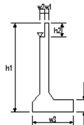
橋台躯体工(4)
