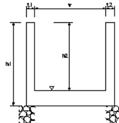
側溝工
