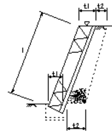
石積(長)工
