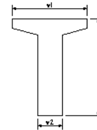
ポストテンション(T)桁製作工
