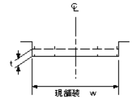
路面切削工
