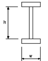
I型プレートガーター 鋼桁補強工(プレートガーター)
