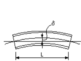
プレビーム用桁製作工 仮組立時 主桁のそり
