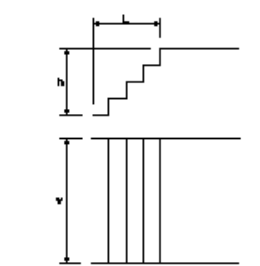
階段工
