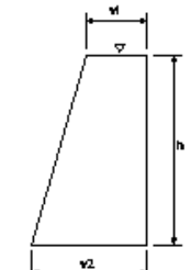
取付擁壁工(1)
