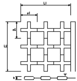
本體工(根固めブロック)
