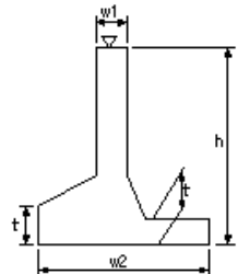
現場打擁壁工(4)
