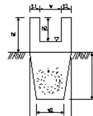
山腹明暗渠工
