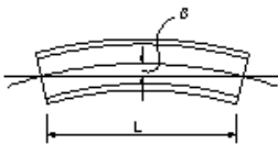
横断歩道橋製作工(主桁、主構のすり)
