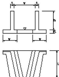
翼壁工
