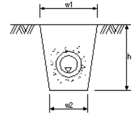
暗渠工
