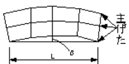
桁製作工(主桁、主構の通り)
