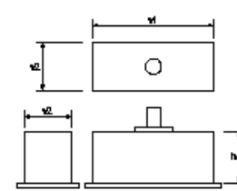
大型標識工(標識基礎工)
