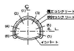
吹付工
