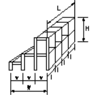
図a 格子形鋼製砂防ダム
