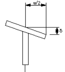
横断歩道橋製作工(フランジの直角度)
