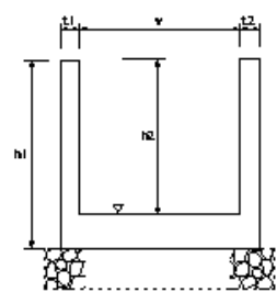
堤脚水路工
