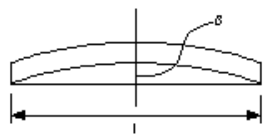
鋼筋補強工(圧縮材の曲がり)
