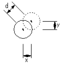
土留・仮締切工(アンカー工) d = \sqrt{x^2 + y^2}
