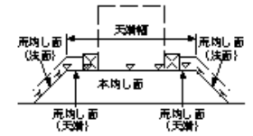
基礎捨石工
