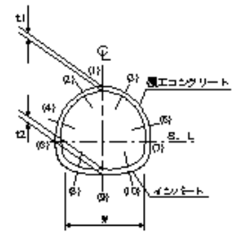
インパート本体内工
