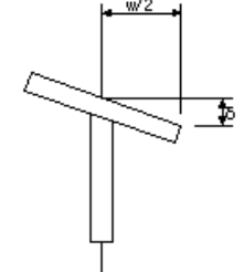
桁製作工(フランジの直角度)
