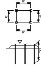
パチカルドレーン工(サンドドレーン工) (ベ ーパドレーン工)(袋詰式サンドドレーン工)
