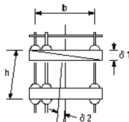
アンカーフレーム製作工
