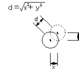
既製杭工
