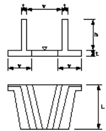
翼壁工・水叩工
