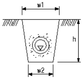
暗渠工
