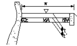
天端被覆工_コンクリート被覆工
