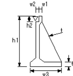
橋台躯体工(2)
