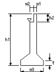
橋台躯体工(3)
