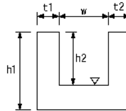
魚道工
