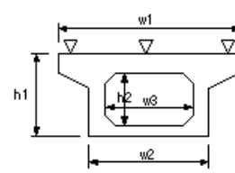
PC箱桁製作工
