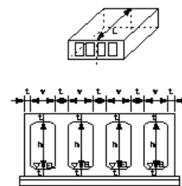
現場打ちボックス工(特殊部)
