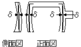
鋼製橋脚製作工(仮組立時)(はりのキャッチャー及び柱の曲がり)
