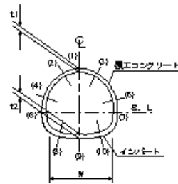
インパート本体内工
