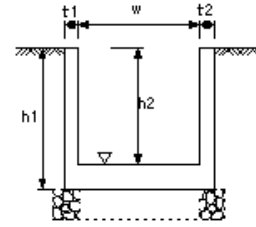
現場打水路工
