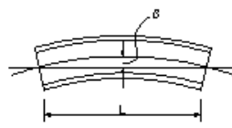
プレビ-ム用桁製作工(主桁のそり)
