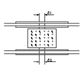
桁製作工(仮組立による検査を省略する場合)(現場継手部のすき間)
