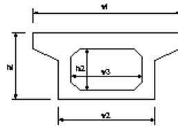
PC押し箱桁製作工
