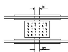
桁製作工(現場継手部のすき間)
