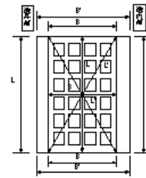
ケーソン製作工(3)
