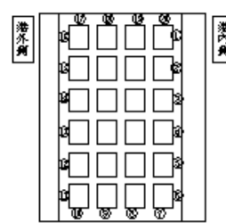
ケーソン製作工(2)
