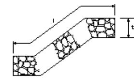
かご工(じゃかご工)
