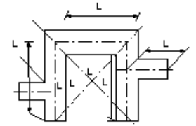
鋼製橋脚製作工(仮組立時)(柱の中心間隔、対角長)
