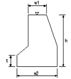
現場打擁壁工(2)
