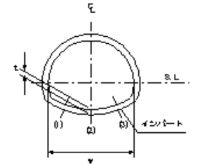
インパート本体工
