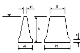
RC躯体工(重力式)(半重力式)
