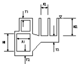
ポンプ場・終末処理場[池・槽]の主構造部
