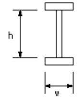
I型鋼げた プレビーム用桁製作工(フランジ幅、腹板高)
