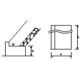
護岸基礎工/場所打コンクリート工
