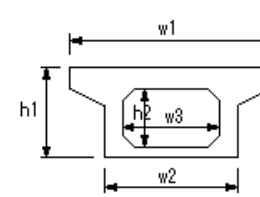
PC押し箱桁製作工
