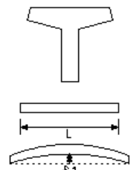
プレビーム用桁製作工(購入工)けた橋立検査省略
