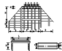
木造橋(上下部構造)
