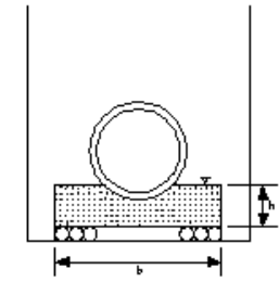
コンクリート基礎
