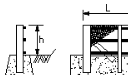
落石防護柵工
