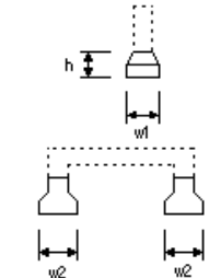
橋脚フーチング工(門型)
