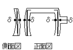
鋼製橋脚製作工(仮組立時)(はりのキャンバー及び柱の曲がり)
