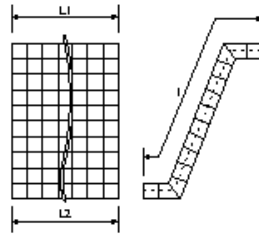
土留・仮締切工(連節ブロック張工)
