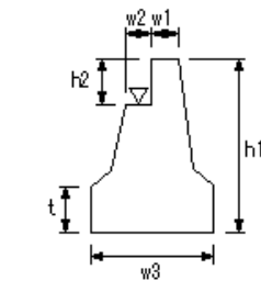
橋台躯体工(1)
