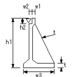
橋台躯体工(2)
