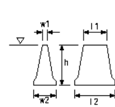
RC躯体工(重力式)(半重力式)
