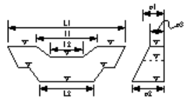
コンクリート堰堤本体工
