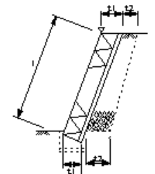
図c 鋼製スリットダムB型
