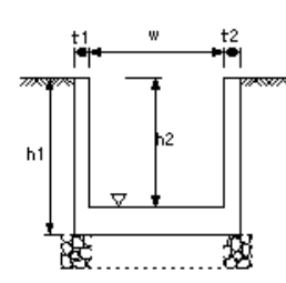
現場排水路工
