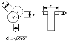
集水井工
