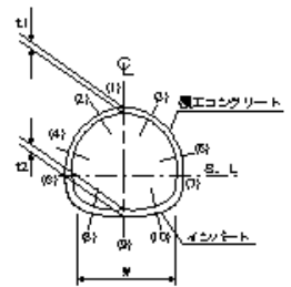
インパート本體工
