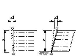
補強土壁工
