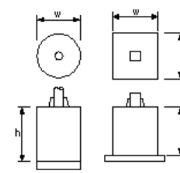
照明工(照明柱基礎工)
