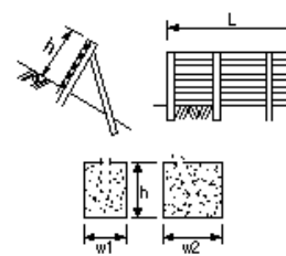
雪崩予防柵工
