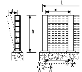
遮音壁本体工
