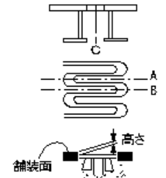
舗装面 expansion device work (鋼製フィンガージョイント)
