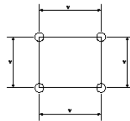
パーチカルドレーン工(サンドドレーン工) (ペーパードレーン工)(袋詰式サンドドレーン工) 固結工(粉体噴射攪拌工)(高圧噴射攪拌工)(セメントミルク攪拌工)(生石灰バ...
