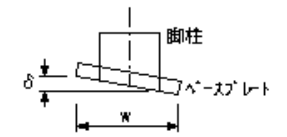
鋼製橋脚製作工(部材)(脚柱とベースプレートの鉛直度)
