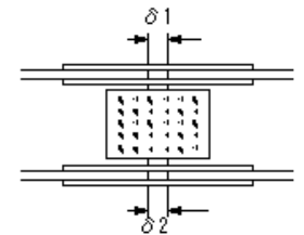
架設工(鋼橋)現場継手部のすき間(仮組立検査省略)
