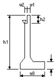
橋台躯体工(4)
