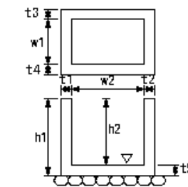
ハンドホール工
