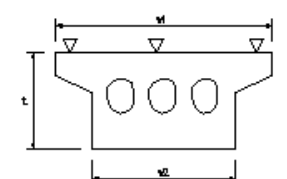
PCホーラスラブ製作工・RC場所打ホーラスラブ製作工・PC版桁製作工
