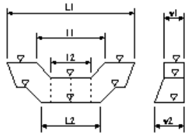
本堤工
