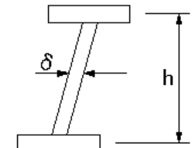
横断歩道橋製作工(主桁、主桁の鉛直度)
