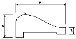
堰本体工・土砂吐工・水叩工
