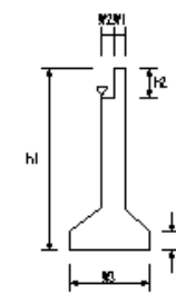
管理橋橋台工(3)
