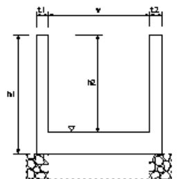
現場水路工
