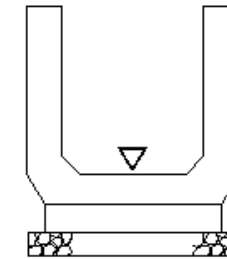
側溝工(プレキャストU型側溝)
