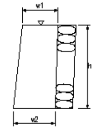
取付擁壁工(3)
