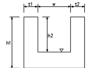
魚道工
