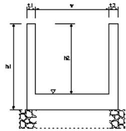
堤脚水路工
