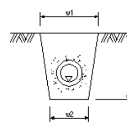
暗渠工(コルゲートパイプ)(ダクタイル铸铁管)
