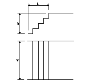
階段工
