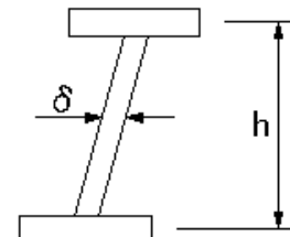
桁製作工(主桁、主構の鉛直度)
