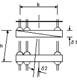
アンカーフレーム製作工
