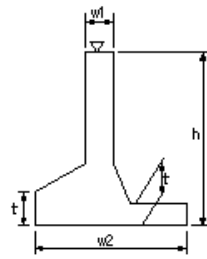
コンクリート擁壁工(4)
