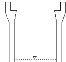
側溝工(自由勾配側溝)
