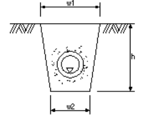
山腹暗渠工
