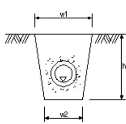
地下排水工
