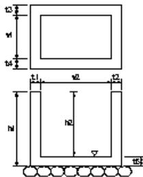
集水枳工
