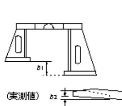
鋼製伸縮継手製作工(仮組立時)
