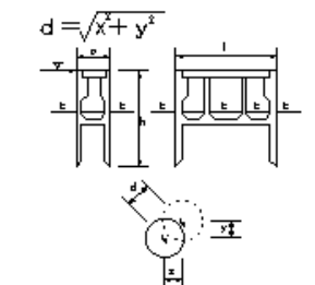
8 ニューマチックケーソン基礎工
