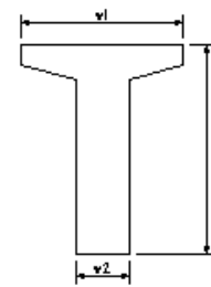
ポストテンションT(①)桁製作工
