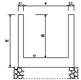
側溝工
