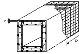
鉄筋の組立て
