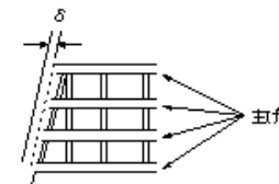
横断歩道橋製作工(主桁、主桁の橋端における出入差)
