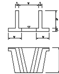
水叩工
