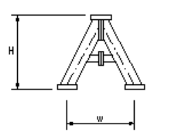
図b 鋼製スリットダムA型
