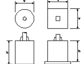
照明工(照明柱基礎工)
