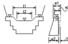
鋼製ダム本体工(不透過型)
