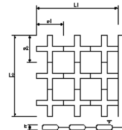
消波ブロック工
