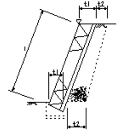
石積(張)工
