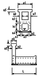
函渠工(本体工)
