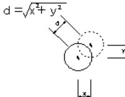
4 既製杭工
