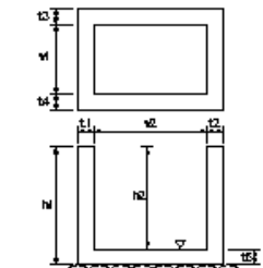
集水樹工
