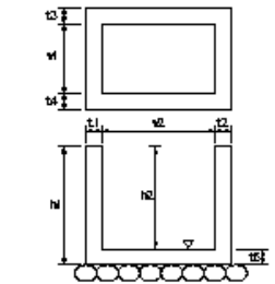
ハンドホール工
