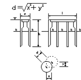
7 オープンケーソン基礎工
