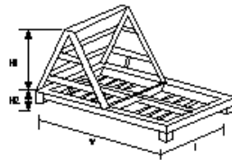
図d 鋼製型スリットダム 鋼製堰堤本体工(透過型)(図d)
