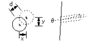
集排水ポーリング工
