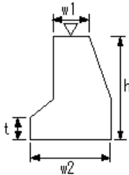
場所打擁壁工(2)
