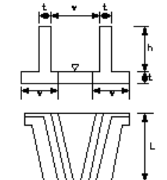
翼壁工・水叩工
