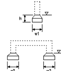
橋脚フーチング工(門型)
