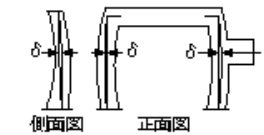
鋼製橋脚製作工(仮組立時)(はりのキヤンバー及び柱の曲がり)
