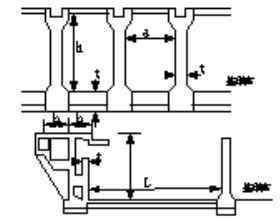
池・槽の主構造部
