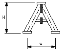
図b 鋼製スリットダムA型
