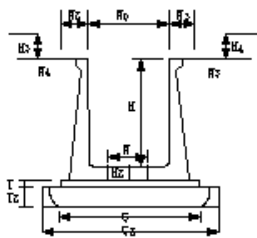
既製品U型水路工
