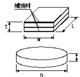
鑄造費(大型ゴム支承工)
