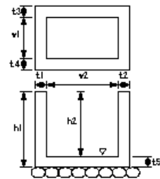
ハンドホール工
