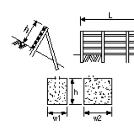
雪崩予防柵工
