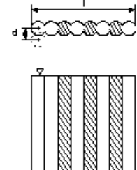
地中連続壁工(柱列式)
