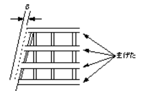
桁製作工(主げた、主構の橋端における出入差)
