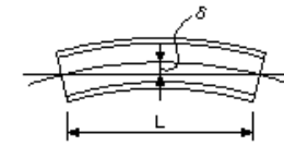
架設工(鋼橋)そり
