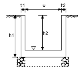
現場打水路工
