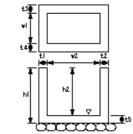
ケーブル配管工(ハンドホール)
