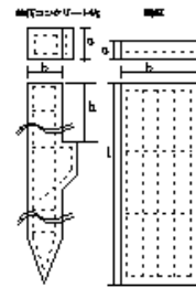
コンクリート板柵
