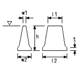
RC躯体工(重力式)(半重力式)
