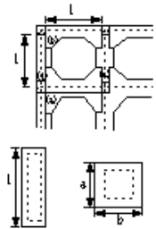
法枠ブロック及び巾杭
