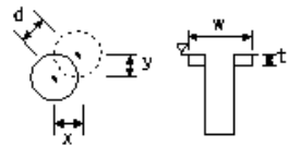
図c 鋼製スリットダムB型 鋼製堰堤本体工(透過型)(図c)
