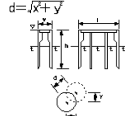
オープンケーソン基礎工
