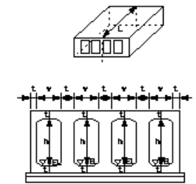
現場打ちボックス工(特殊部)
