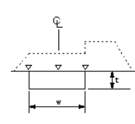
路床安定処理工
