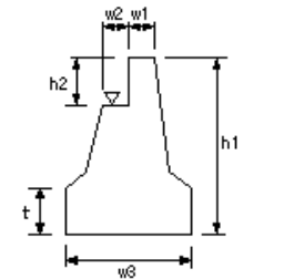
管理橋橋台工(1)
