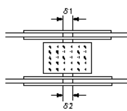
桁製作工(現場継手部のすき間)
