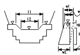
鋼製堰堤本体工(不透過型)
