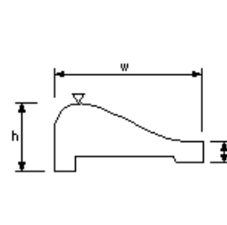
堰本体工・水叩工・土砂吐工
