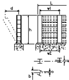
遮音壁本体工
