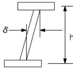
架設工(鋼橋)主げた、主構の鉛直度(仮組立検査省略)
