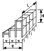
図a 格子形鋼製砂防ダム
