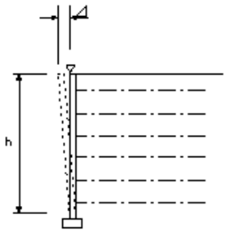
補強土壁工(補強土(テールアルメ)壁工) (多数アンカー式補強土工法)
