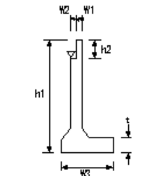
管理橋橋台工(4)
