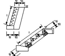
コンクリートブロック工(コンクリートブロック積)(コンクリートブロック張り)
