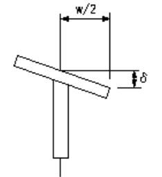
プレビーム用桁製作工(フランジの直角度)
