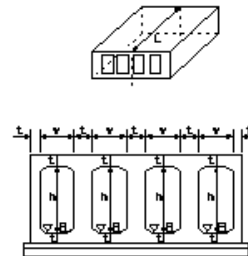
現場打躯体工
