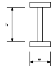
I型鋼(材) プレビーム用桁製作工(I型鋼けた)
