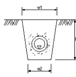
管渠工
