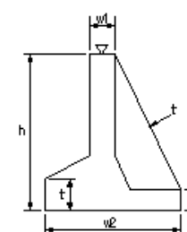
取付擁壁工(5)
