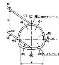
覆工コンクリート工・側壁コンクリート工
