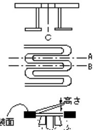
伸縮装置工(鋼製フィンガージョイント)
