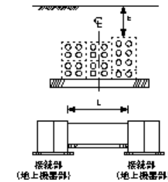
管路工
