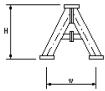
図b 鋼製スリットダムA型
