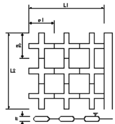
本體工(根固めブロック)
