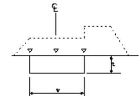
路床安定処理工
