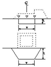
置換工
