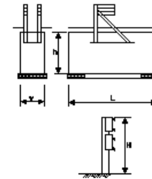
路側防護柵工(ガードケーブル)
