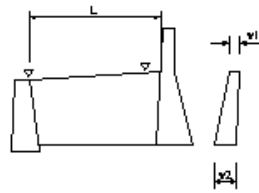
側壁工
