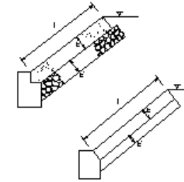
護岸工_コンクリート被覆工
