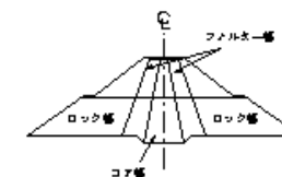
フィルターの盛立
