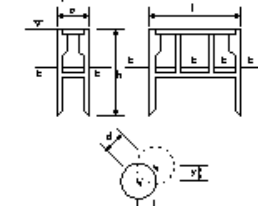
ニューマチックケーソン基礎工
