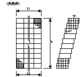
ふとんかご、かご枠
