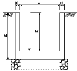
場所打水路工
