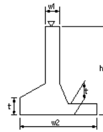
場所打擁壁工(4)
