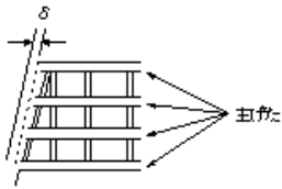
横断歩道橋製作工(主桁、主構の橋端における出入差)
