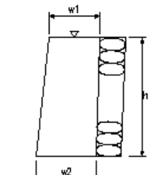
コンクリート擁壁工(3)
