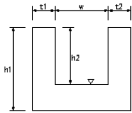
魚道本體工
