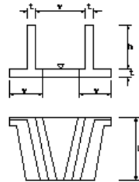
翼壁工
