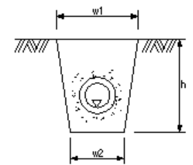
暗渠工
