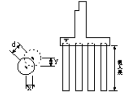
深礎工
