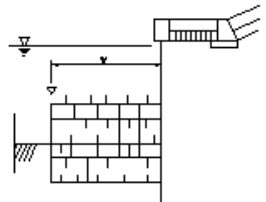
沈床工
