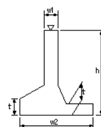
取付擁壁工(4)
