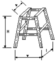
図c 鋼製スリットダムB型
