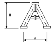
図b 鋼製スリットダムA型
