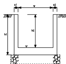
側溝工
