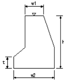
場所打擁壁工(2)
