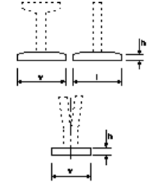
橋脚フーチング工(型・T型)
