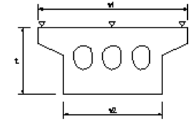
PC木口スラブ製作工
