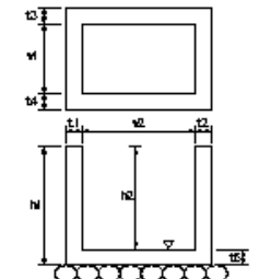
集水桝・マンホール工
