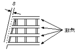
架設工(鋼橋)主げたの橋端における出入差
