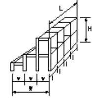
図a 格子形鋼製砂防ダム
