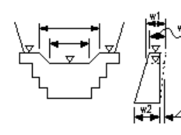
鋼製堰堤本体工(不透過型)
