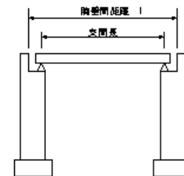
橋台躯体工(胸壁間距離及び支間長)
