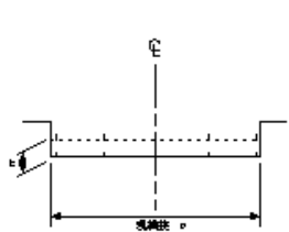
路面切削工
