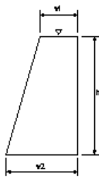
取付擁壁工(1)
