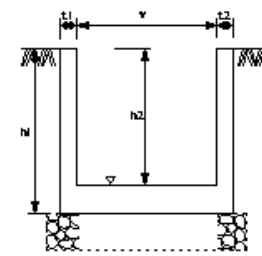
側溝工
