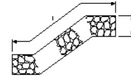
じゃかご
