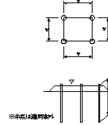
パーティカルドレーン工(サンドドレーン工)(ペーパードレーン工)(袋詰式サンドドレーン工)
