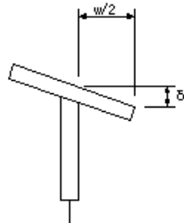
プレビーム用桁製作工(フランジの直角度)
