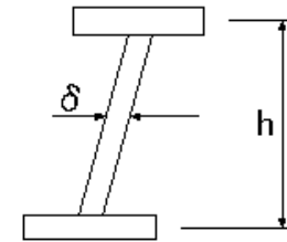
架設工(鋼橋)主げた、主構の鉛直度
