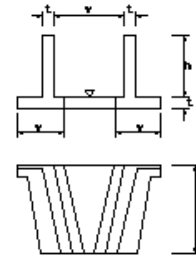
水叩工
