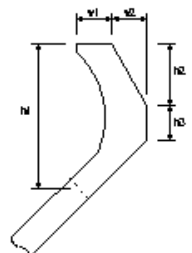
波返工
