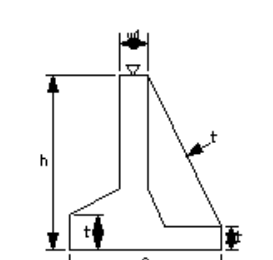
取付擁壁工(5)
