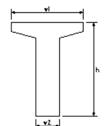
ポストテンション(D)桁製作工
