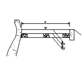
天端被覆工_コンクリート被覆工
