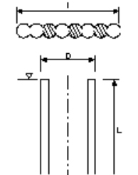
地中連続壁工(柱列式)
