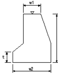
取付擁壁工(2)
