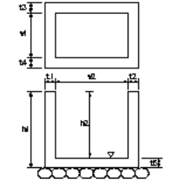
ケーブル配管工(ハンドホール)
