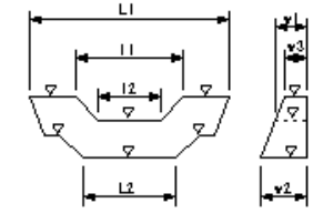
床固め本体工
