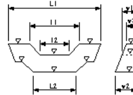
コンクリートダム本体工・コンクリート副ダム工
