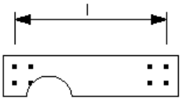
桁製作工(部材長)(プレートガーター)
