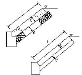
護岸工/裏法被覆工_コンクリート被覆工
