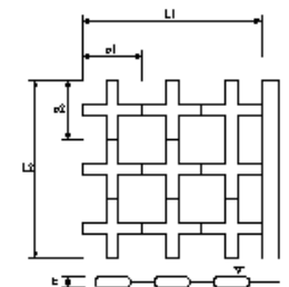
水叩工(根固めブロック)
