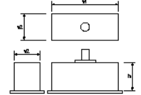
大型標識工(標識基礎工)
