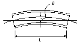
横断歩道橋製作工(主桁、主構のそり)
