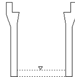
側溝工(自由勾配側溝)
