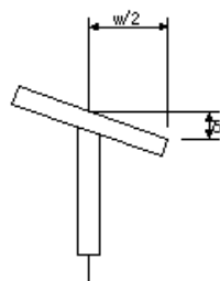
部材 プレベーム用桁製作工(フランジの直角度)
