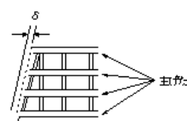
桁製作工 (主桁、主構の橋端における出入り差)
