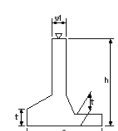
取付擁壁工(4)
