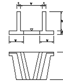
水叩工
