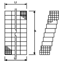
かご工(ふとんかご工)
