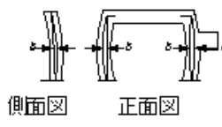
鋼製橋脚製作工(仮組立時)(はりのキャンバー及び柱の曲がり)
