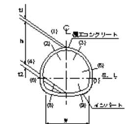
インパート本体内工
