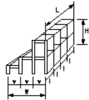
図a 格子形鋼製砂防ダム 鋼製ダム本体工(透過型)(図a)
