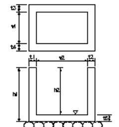
集水桝・マンホール工
