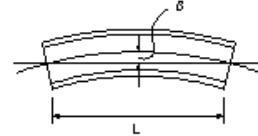
プレビーム用桁製作工(主桁のそり)
