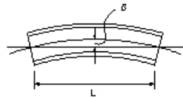
桁製作工(主桁、主構のぞり)
