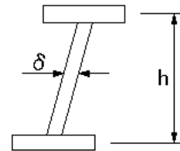
桁製作工 (主桁、主構の鉛直度)
