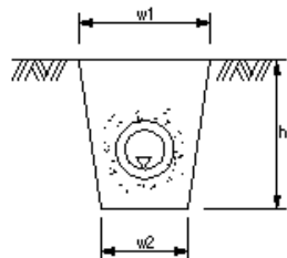
山腹暗渠工
