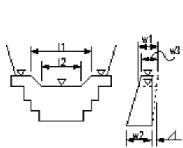
鋼製ダム本体工(不透過型)
