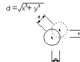
既製杭工
