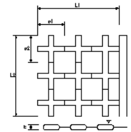
本体工(根固めブロック)
