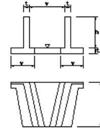
翼壁工
