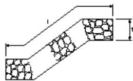
縁切工(ジャかご工)
