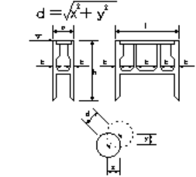
ニューマッチャーケーソン基礎工
