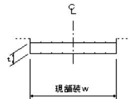
路面切削工
