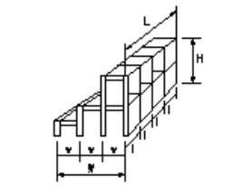
図a 格子形鋼製砂防ダム
