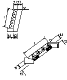
コンクリートブロック工(コンクリートブロック積み)(コンクリートブロック張り)
