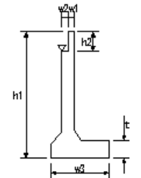
橋台躯体工(4)
