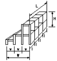
図a 格子形鋼製砂防ダム 鋼製堰堤本体内工(透過型)(図a)
