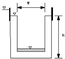
越流せき工
