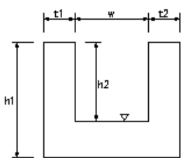
魚道本体工
