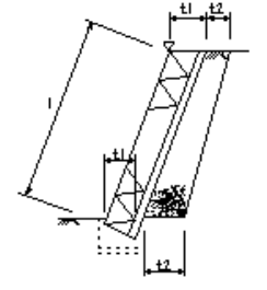
石積(張)工
