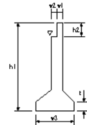
橋台躯体工(3)
