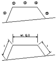
護岸基礎工/突堤基礎工_捨石工
