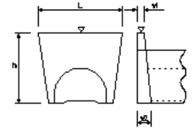
坑門本体工
