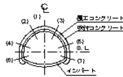
吹付工
