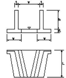
水叩工
