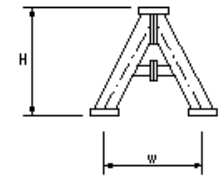
図b 鋼製スリットダムA型 鋼製堰堤本体内工(透過型)(図b)
