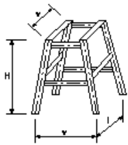
図c 鋼製スリットダムB型 鋼製堰堤本体内工(透過型)(図c)
