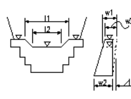
鋼製堰堤本体内工(不透過型)
