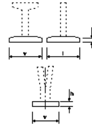
橋脚フーチング工(型)(T型)
