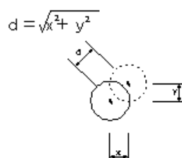
既製杭工(既製コンクリート杭)(鋼管杭)(H鋼杭)
