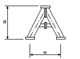
図b 鋼製スリットダムA型
