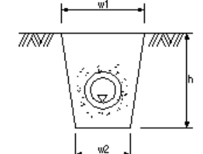
山腹暗渠工
