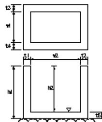
集水樹工
