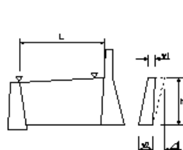
鋼製側壁工
