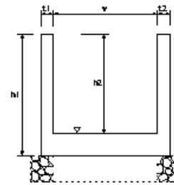
現場打水路工
