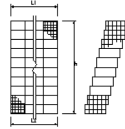
羽口工(ふとんかご)(かご枠)
