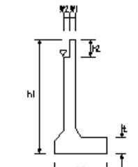
管理橋橋台工(4)
