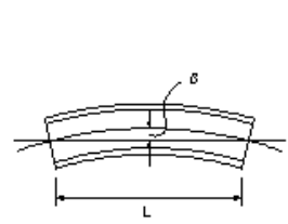
プレビーム用桁製作工(主桁のそり)
