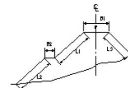
盛土
