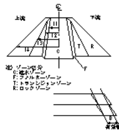
堤体盛土
