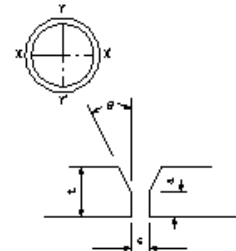
V型開先(片面溶接)
