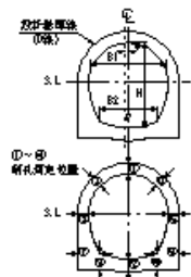
水路トンネル(コンクリート覆工)
