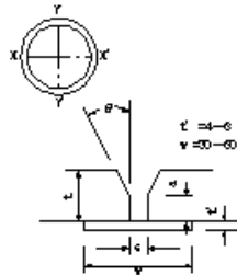
V型開先(片面裏当溶接)
