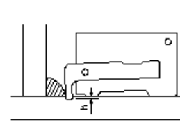
すみ肉溶接(アングカット)
