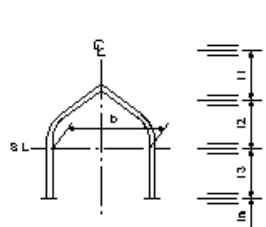
水路トンネル(支保工)
