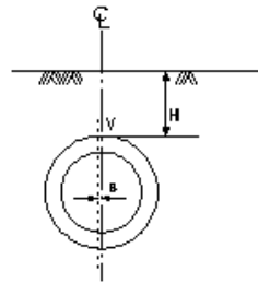
管水路(硬質塩化ビニル管)
