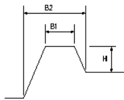
畦畔工
