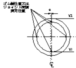
管水路(コンクリート二次製品)_RC管
