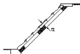
石張工 ブロック張工
