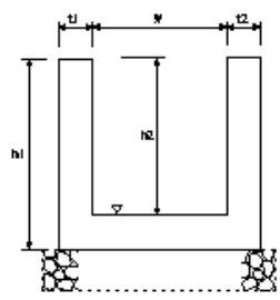
開水路(現場打)
