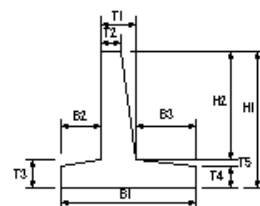
コンクリート擁壁
