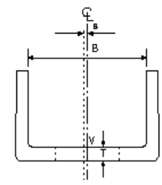
コンクリート二次製品水路 コンクリート二次製品大型フリューム水路 鉄筋コンクリート...
