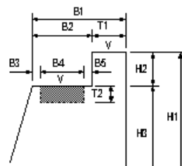
橋台各部
