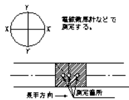
アスファルト塗覆装
