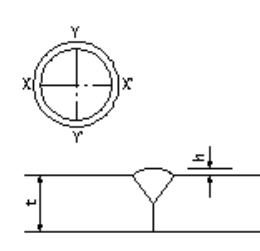
周継手溶接(余盛高)
