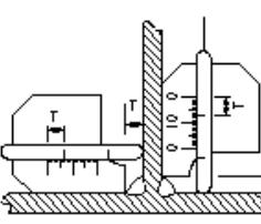
すみ肉溶接(脚長)
