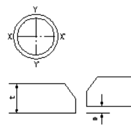
周継手溶接(目違い)
