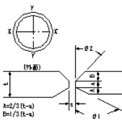
X型開先(両面溶接)
