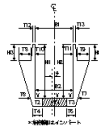
洪水吐
