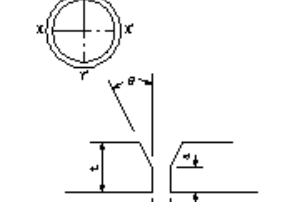
V型開先(両面溶接)
