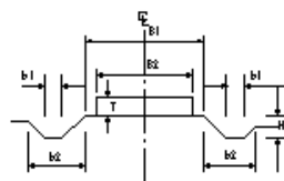
道路工(耕作道)
