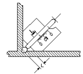
すみ肉溶接(のど厚)
