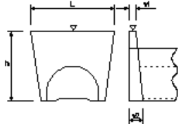
坑門本体工
