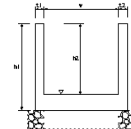
場所打水路工
