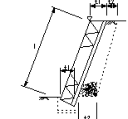
石積(張)工
