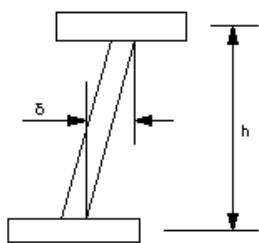
横断歩道橋製作工(主桁、主構の鉛直度)
