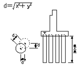
深礎工
