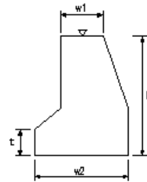
取付擁壁工(2)
