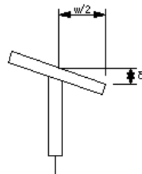
プレベーム用桁製作工(フランジの直角度)
