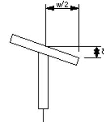
桁製作工(仮組立による検査を省略する場合)(フランジの直角度)
