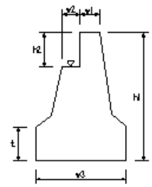
橋台躯体工(1)
