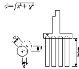
場所打杭工
