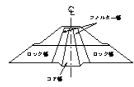
コアの盛立
