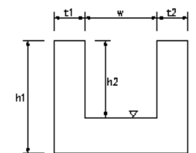
魚道本体工
