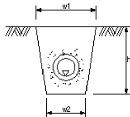
暗渠工
