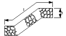
かごマット
