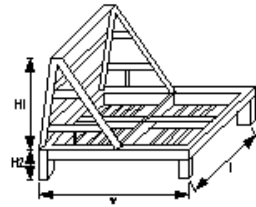
図d 鋼製L型スリットダム 鋼製堰堤本体工(透過型)(図d)
