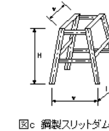
図c 鋼製スリットダムB型
