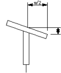
横断歩道橋製作工(仮組立による検査を省略する場合)(フランジの直角度)
