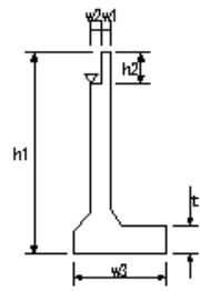
橋台躯体工(4)
