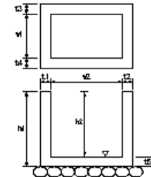
集水栴工
