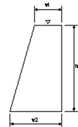
取付擁壁工(1)
