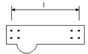
横断歩道橋製作工(仮組立による検査を省略する場合)(部材長)(鋼けた)
