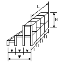
図a 格子形鋼製砂防ダム 鋼製堰堤本体工(透過型)(図a)
