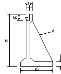
橋台躯体工(2)
