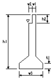
橋台躯体工(3)
