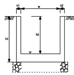
側溝工
