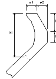
波返工
