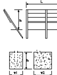
防雪柵工
