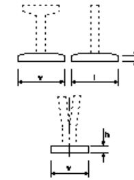
橋脚ワーチング工(型・T型)
