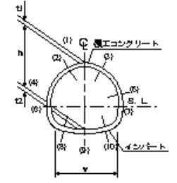
覆工コンクリート工・側壁コンクリート工
