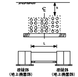
管路工
