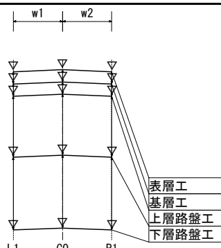
測定箇所図
